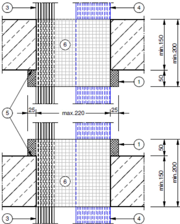
Schnitt Decke - unterseitige Aufdopplung
