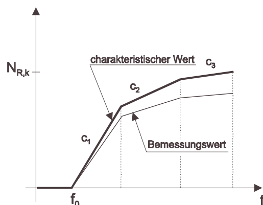
Bild 1: Federkennlinie (sinngemäß)
