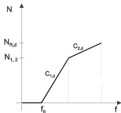
Bild 2: trilineare Federkennlinie
