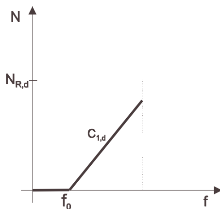
Bild 1: bilineare Federkennlinie
