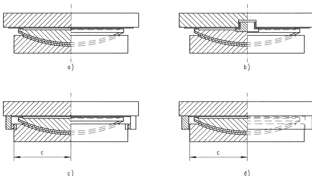
Abb. A.2 — MAURER MSM® Kalottenlager
