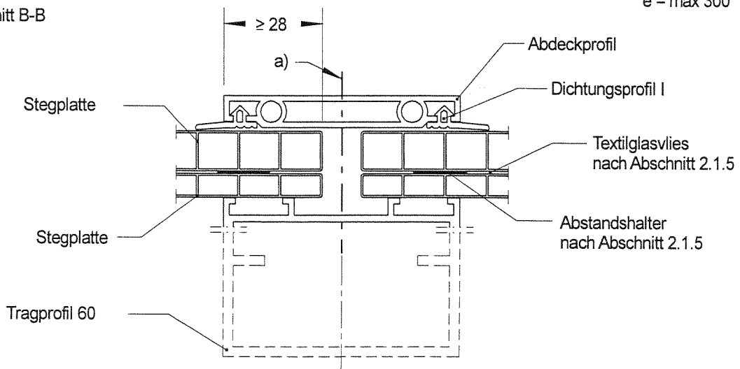
Schnitt C-C
