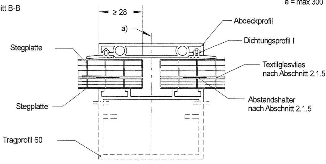
Schnitt C-C
