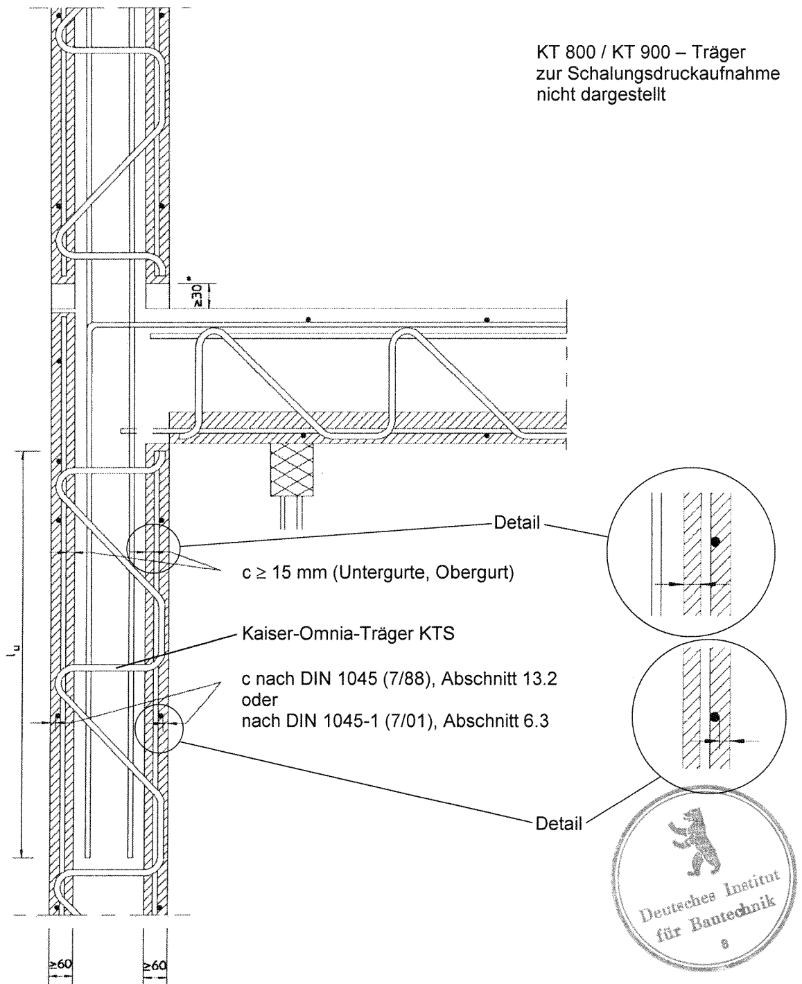
Bild 13 Deckenanschluss bei bewehrter Wand auch nicht vorwiegend ruhende Belastung, biegesteifer Anschluss
