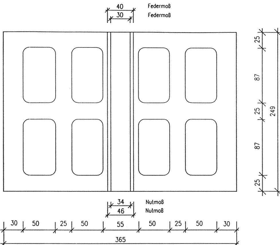
Stirnseiten-Ansicht
