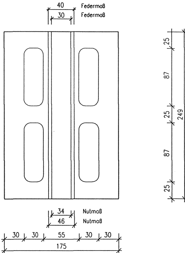
Stirnseiten-Ansicht
