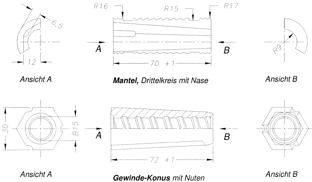
Bild 2: Einzelteile und Abmessungen
