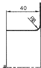
Detail F Anschlußstutzen
