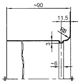
Detail E Anschlußstutzen
