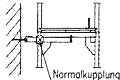
Schnellanker
