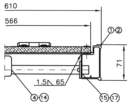
Schnitt B-B
