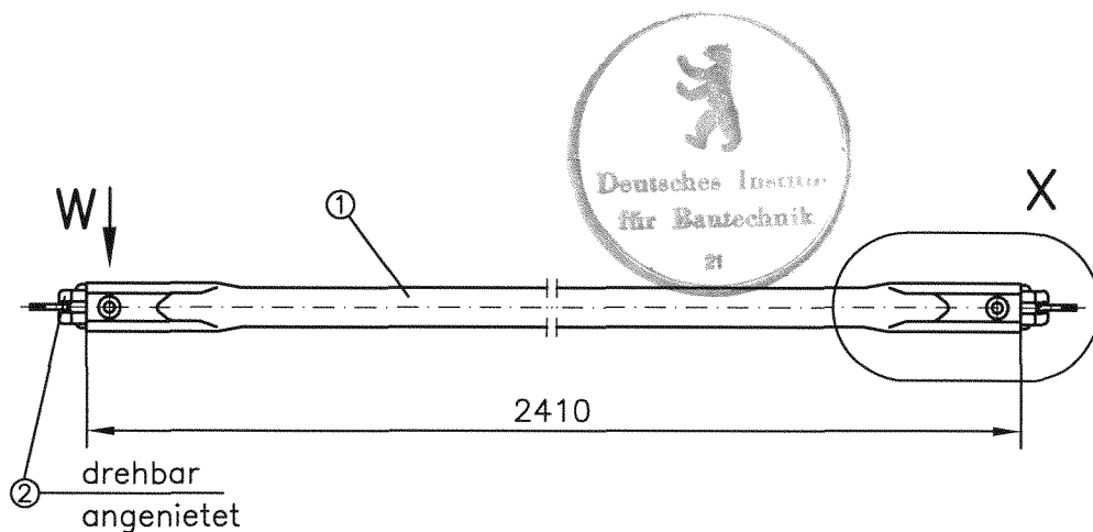
Ansicht W
