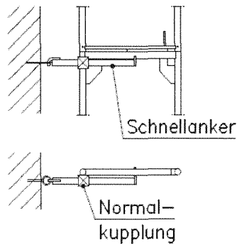
Bild 2b: Schnellanker
