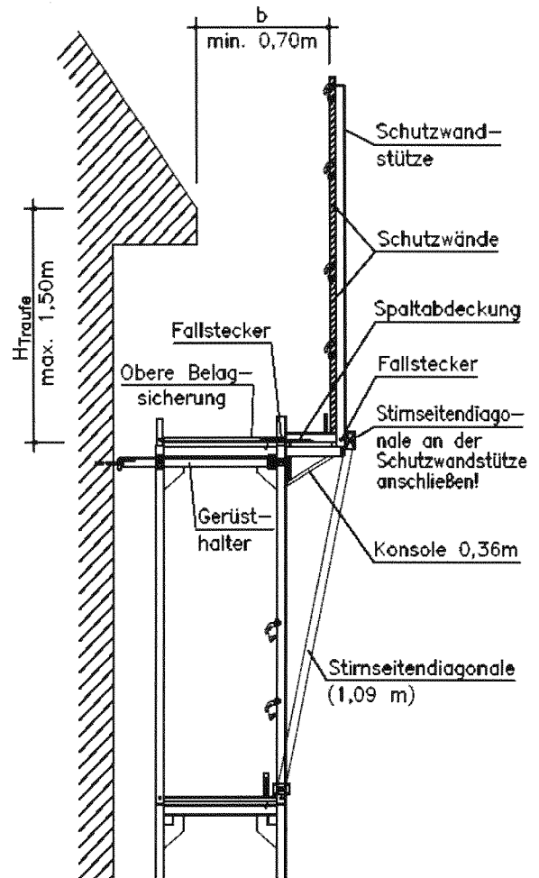
Bild 5b: Schutzwand auf Konsole 0,36 m
