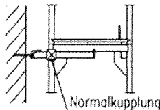
Schnellanker
