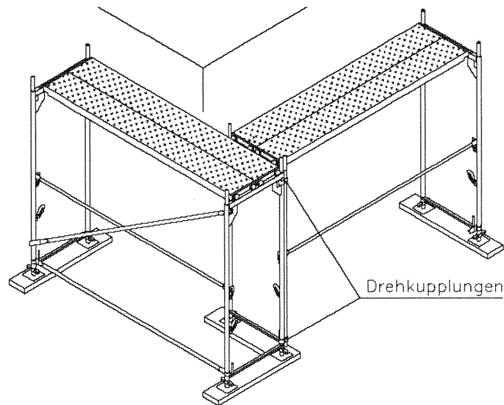
Bild 3a: Eckausbildung mit Drehkupplungen (Gerüstverankerung nicht dargestellt)
