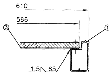
Schnitt B-B
