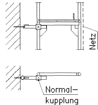
Bild 2c: Gerüsthalter
