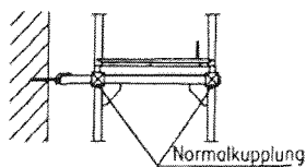
Gerüsthalter
