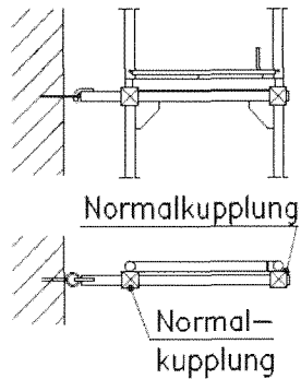
Bild 2a: Gerüsthalter
