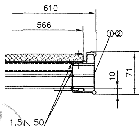
Schnitt A-A
