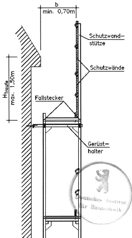
Bild 5a: Dachfangergerüst
