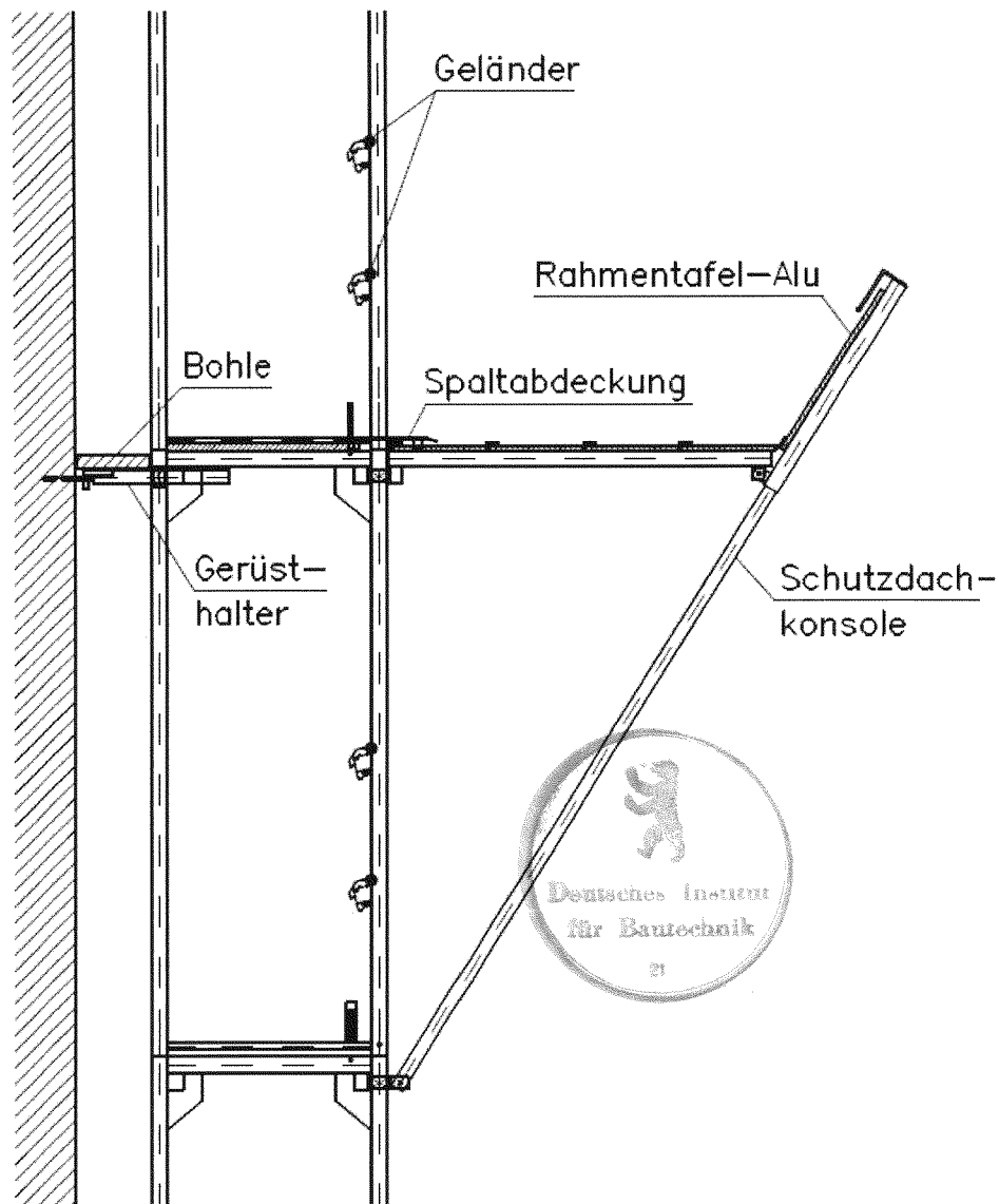
Bild 6: Schutzdach mit Schutzdachkonsolen
