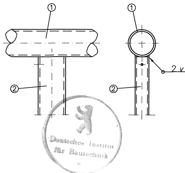
Detail Y
