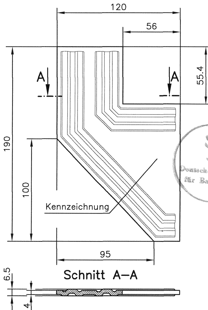
④ Knotenblech \equiv 190 \times 4 S235JR, DIN EN 10025-2
