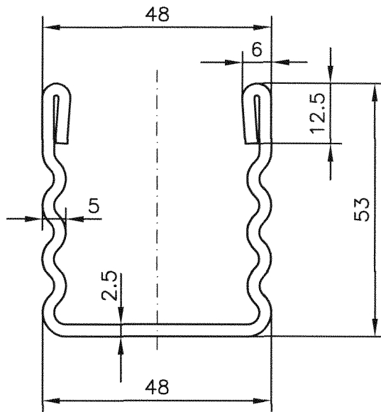
③ Kopfriegel U-Profil, gewellt 53x48x2.5 S235JR, R_{eH} \geq 320 \text{ N/mm}^2 , DIN EN 10025-2
