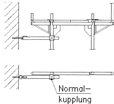
Bild 2e: Gerüsthalter
