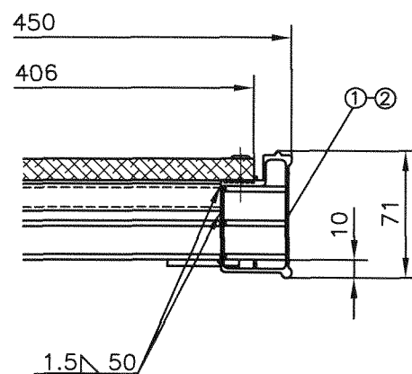
Schnitt A-A
