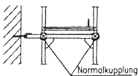
Gerüsthalter
