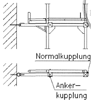
Bild 2d: Gerüsthalter
