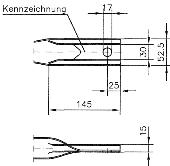
Detail X ohne Pos. ②
