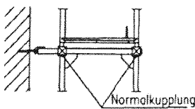
Gerüsthälter
