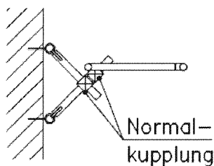
Bild 2h: V-Anker
