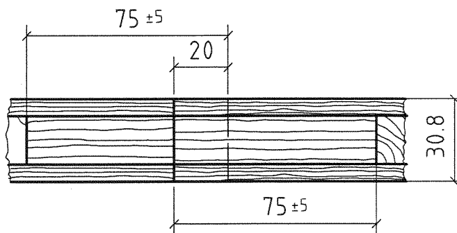
Keilzinkenlängsverbinding im Gurt und Steg Keilzinkenverbinding I 20 DIN68140
