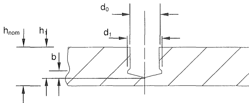
2. Bohrlochgeometrie
