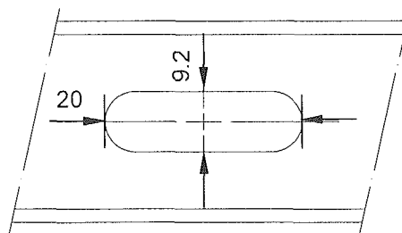
2. Langloch: an Plattentragprofil (Gleitpunkt)
