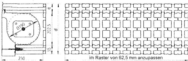
Rollladenkasten „Ri“ (Innenrevision)
