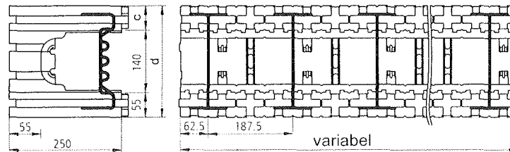
Sturzstein
