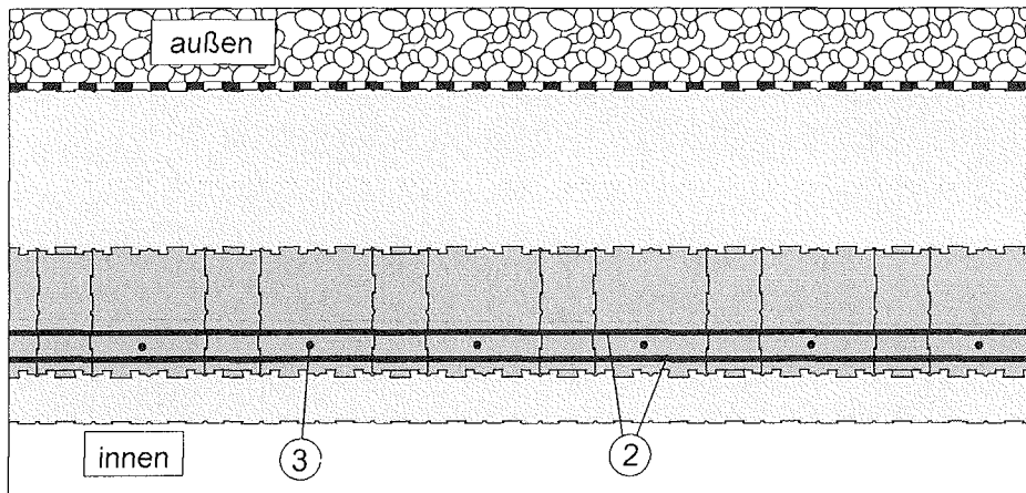
Horizontalschnitt einer Keller-Außenwand mit Darstellung der Bewehrungsanordnung entsprechend den statischen Berechnungen
