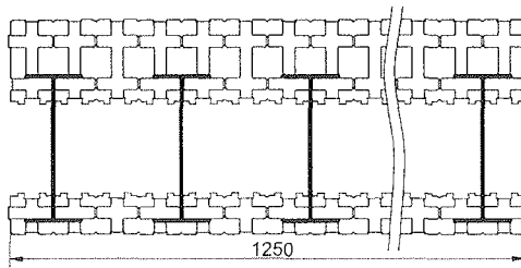
31er-Element
