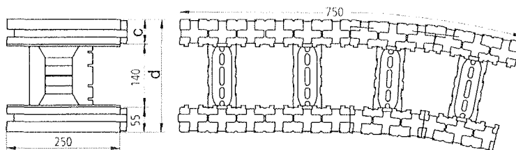
Bogenanschlusselement
