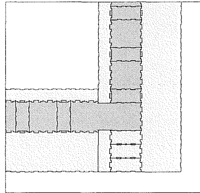
2. Schicht
