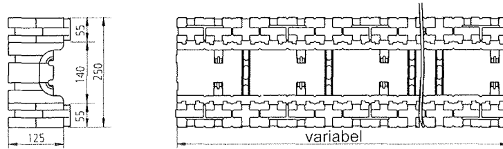
25er-Innentürsturz
