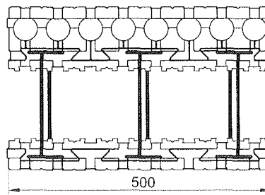
31er-Schalldämmstein
