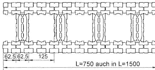
25er-Element
