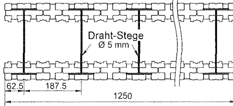
25er-Element
