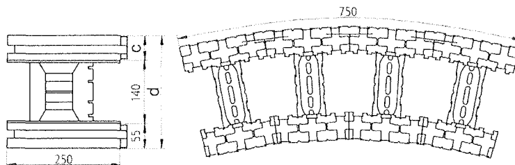
Bogenelement
