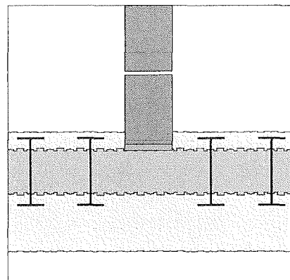
Mauerwerk eingebunden
