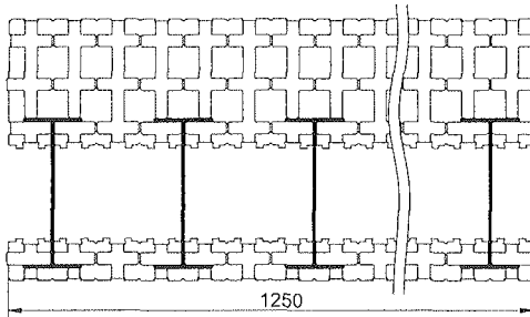
37er-Element
