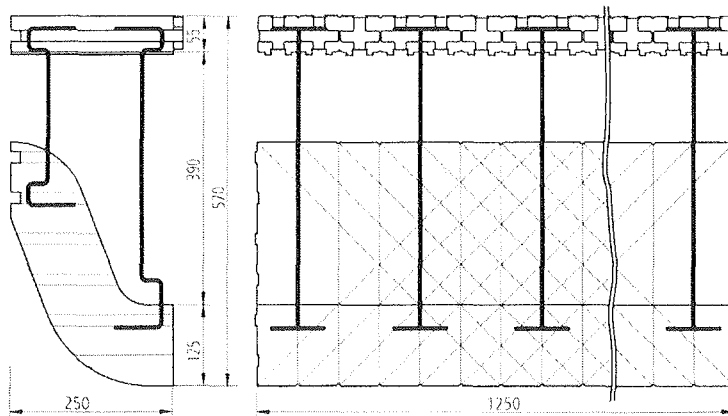
Kragstein
