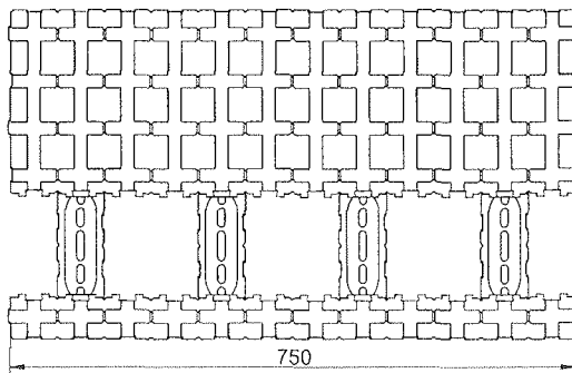
43er-Element
