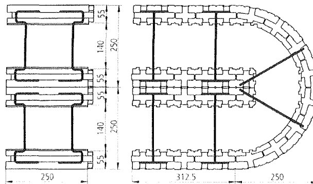
25er-Eckrundstein
