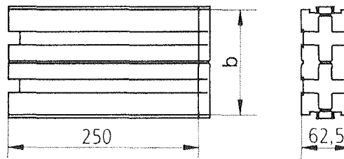
Type 2 / Endstück
