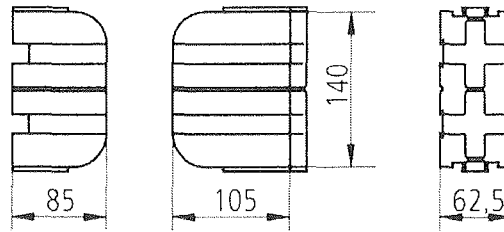
Typ 1 / 140er-Endstück
