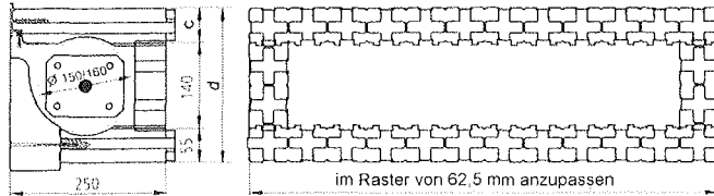
Rollladenkasten „Ri“ (Innenrevision)
