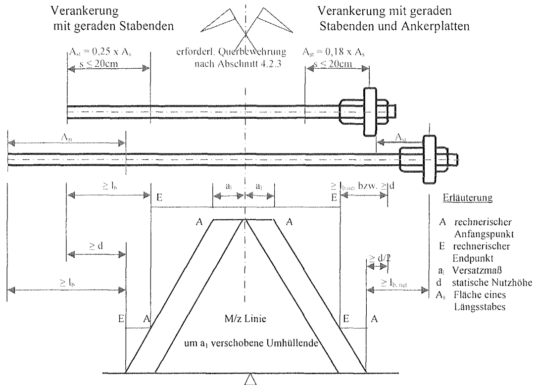
Bild 3b Beispiel für die Verankerung von Stäben d_s = 40 bzw. 50\text{mm} mit geraden Stabenden und Ankerplatten im Stützbereich massiger Bauteile nach Abschnitt 4.2.2 (4) Erforderliche Querbewehrung: A_{st} = 0,18 \times A_s , s \leq 20\text{cm} bzw. nach Abschnitt 4.2.3
