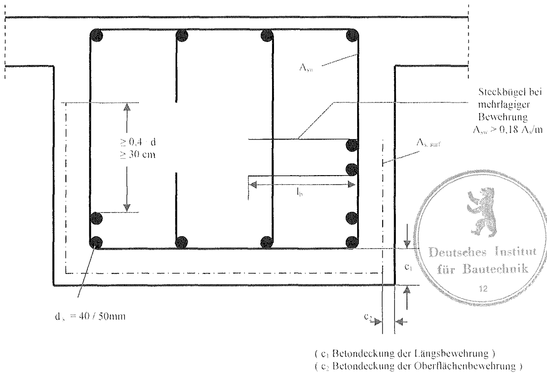
Bild 4b Balken und Anordnung von Steckbügeln bei mehrlagiger Bewehrungen
