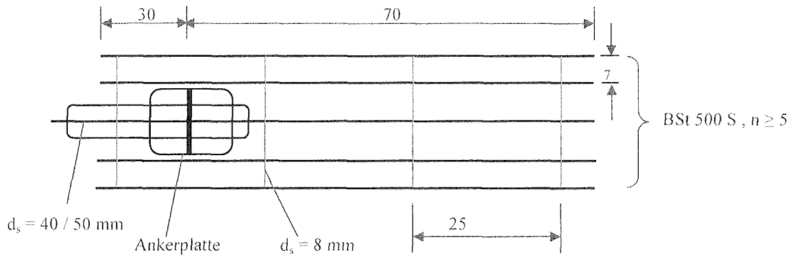
Beispiel für die Rückverankerung von Ankerplatten
