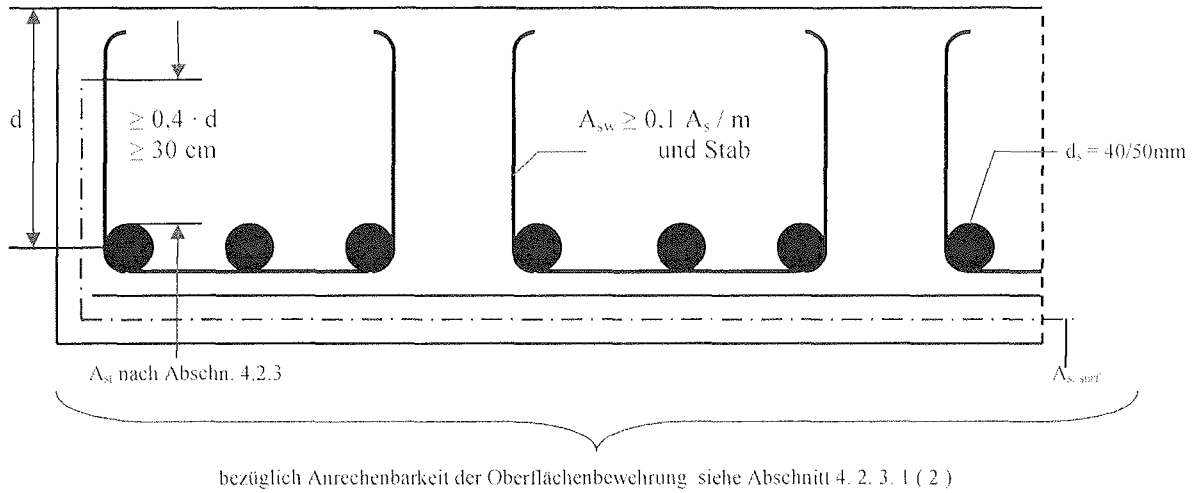
Bild 4b Balken und Anordnung von Steckbügeln bei mehrlagiger Bewehrungen
