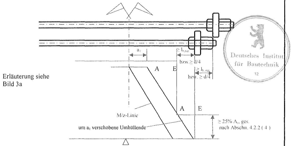
Bild 3b Beispiel für die Verankerung von Stäben d_s = 40 bzw. 50\text{mm} mit geraden Stabenden und Ankerplatten im Stützbereich massiger Bauteile nach Abschnitt 4.2.2 (4) Erforderliche Querbewehrung: A_{st} = 0,18 \times A_s , s \leq 20\text{cm} bzw. nach Abschnitt 4.2.3
