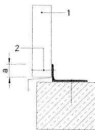
Bild 4 Fußpunkt Wandelement aufgesetzt
