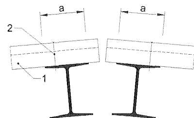
Bild 5 First
