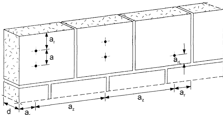
Bild 7: Anordnung der Dübel
