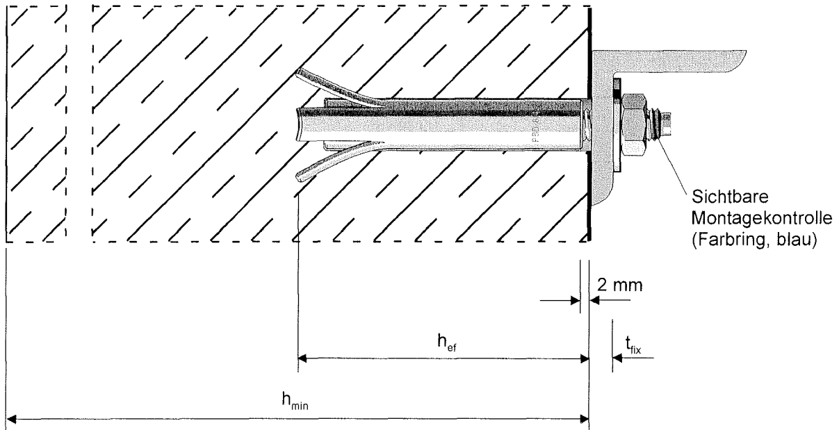
Bild 1: Porenbetondübel HPD, Außengewinde
