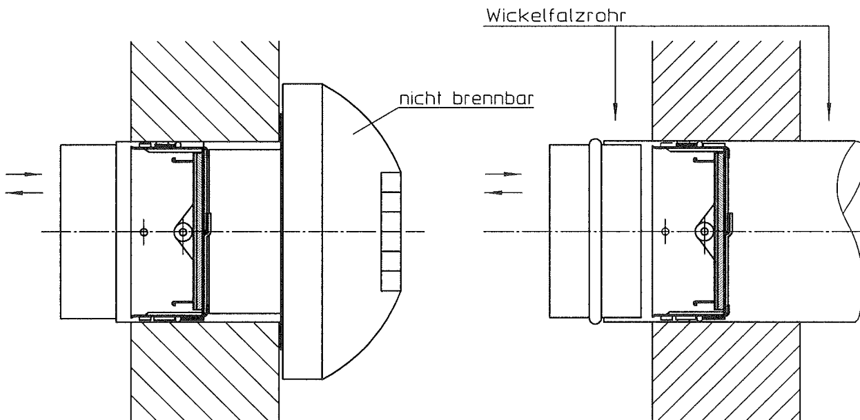
Einbau mit Mauerrahmen oder Wickelfalzrohr und eingestecktem Abluftventil
