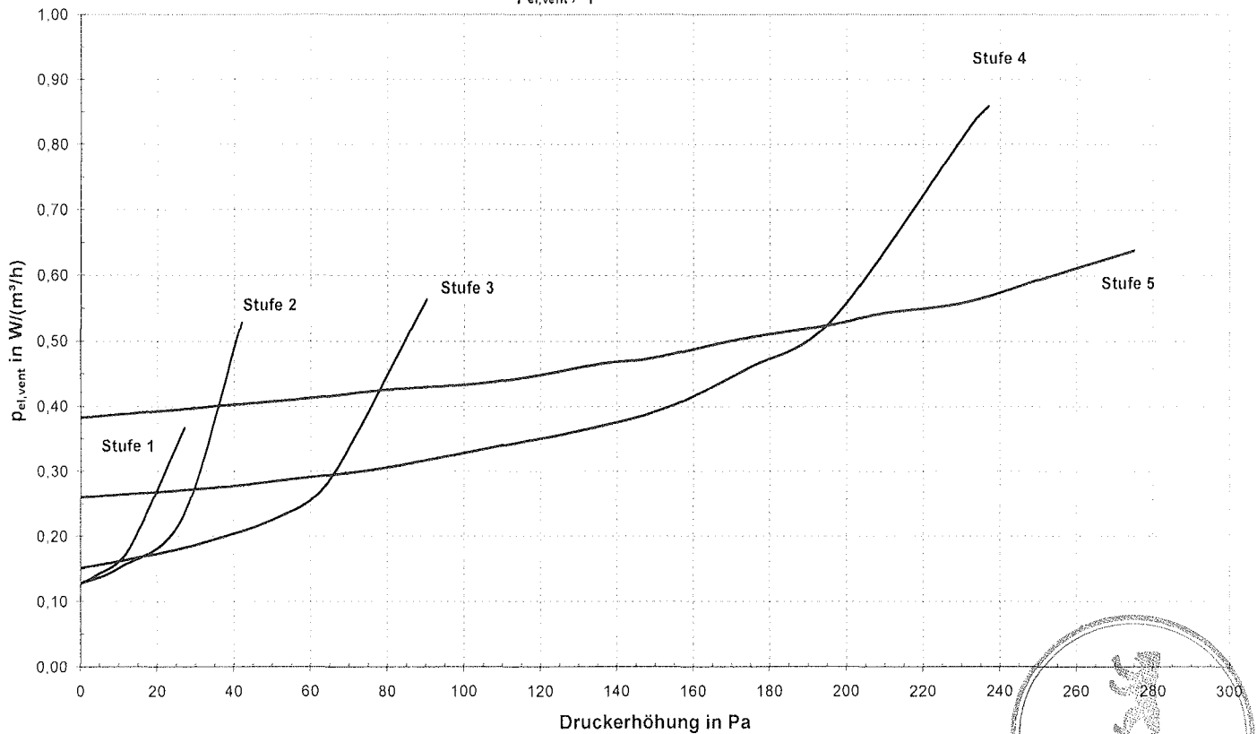
p_{el,vent} , p-Kennlinien AB/FO
