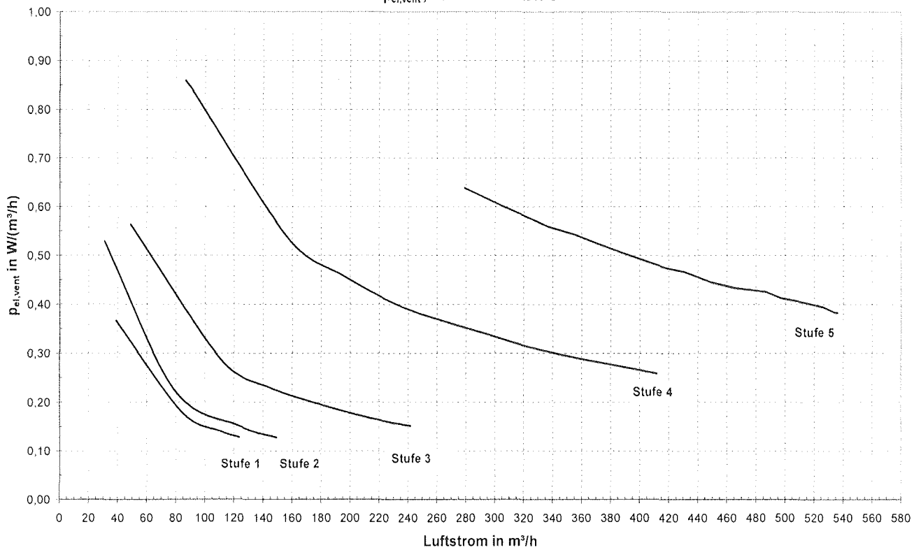
p_{el,vent} , V-Kennlinien AB/FO
