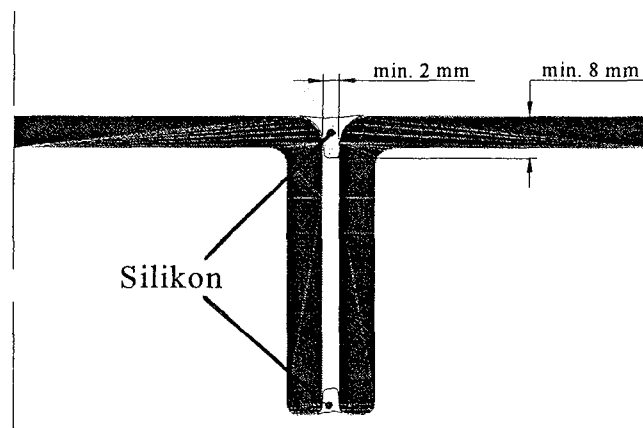
Zeichnung 2: Fugenausbildung bei einschaliger Verglasung mit LINIT-Profilbauglas
