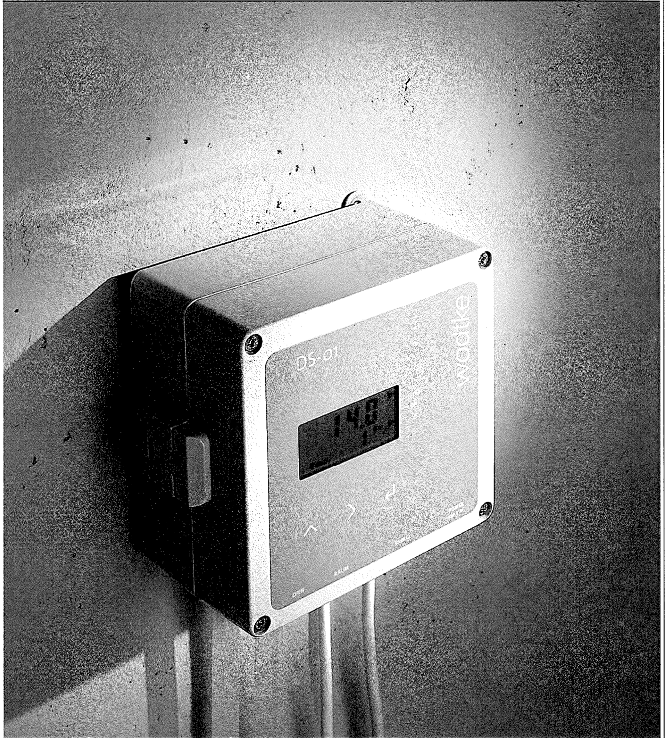
Differenzdruckschalter DS 01:
