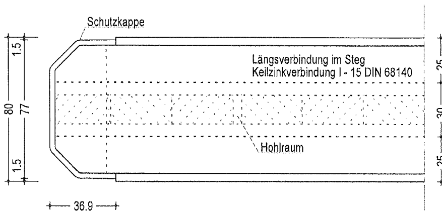
Draufsicht Masstab 1 : 2
