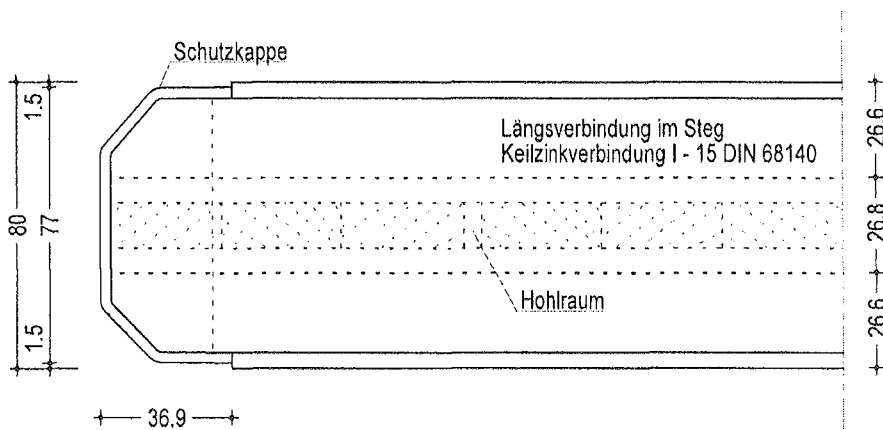
Draufsicht Masstab 1 : 2
