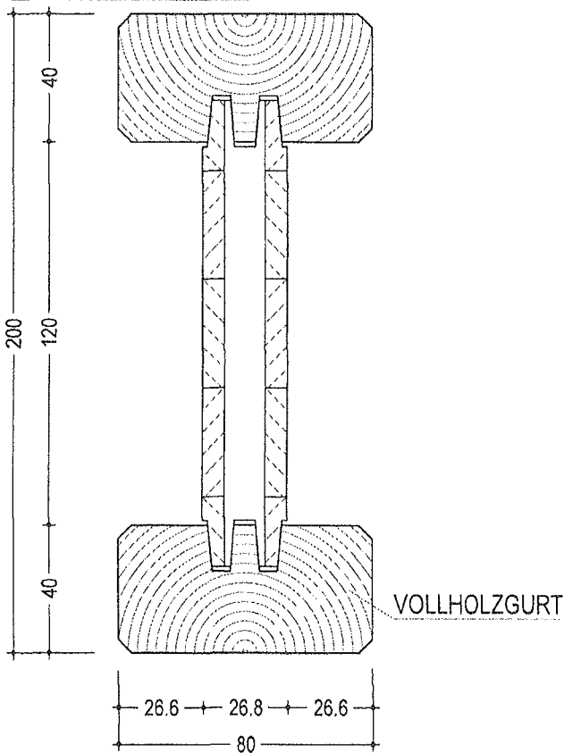
HT 20 Masstab 1 : 2
