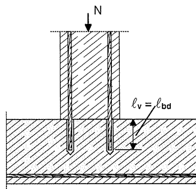
Bild 4: Bewehrungsanschluss überwiegend auf Druck beanspruchter Bauteile. Die Bewehrungsstäbe werden auf Druck beansprucht.
