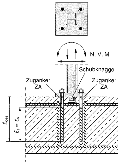
Bild 6: Übergreifungsstoß einer biegebeanspruchten Stütze an ein Fundament
