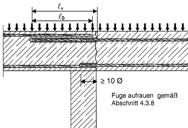
Bild 1: Übergreifungsstoß in Platten und Balken
