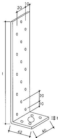
Bild A.7 Typischer Betonflachstahllanker
