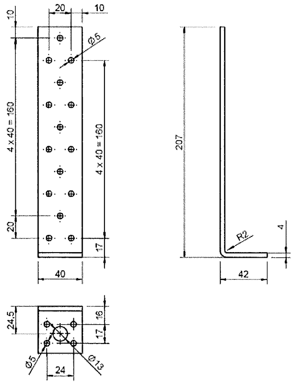
Bild A.4 Maße des Betonflachstahllankers 40 x 200 x 4,00
