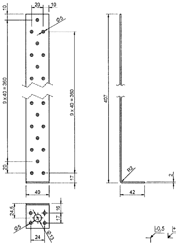
Bild A.3 Maße des Betonflachstahllankers 40 x 400 x 2,00
