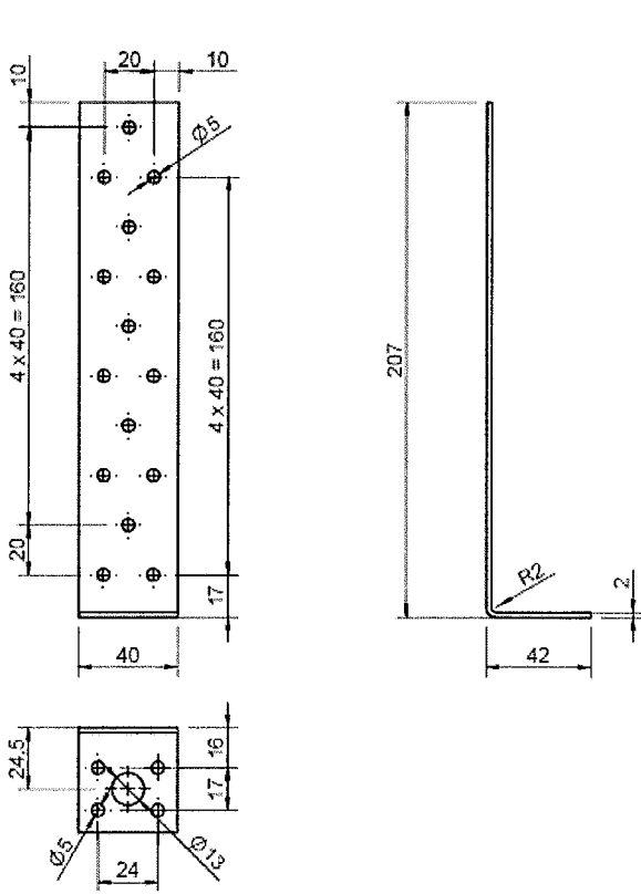
Bild A.1 Maße des Betonflachstahllankers 40 x 200 x 2,00
