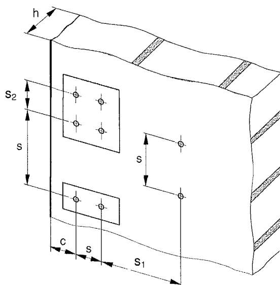
Anordnung der Dübel im Mauerwerk (Nutzungskategorie "b" und "c")
