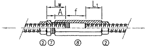
Bild 5 Muffenstoß – Spannschloß Ø12-32
