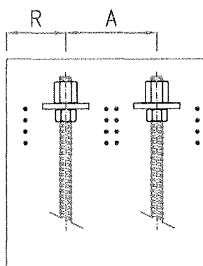
unversetzte Verankerung
