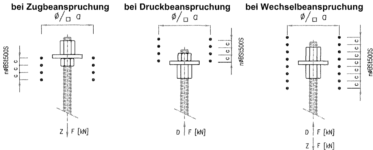
unversetzte Verankerung
