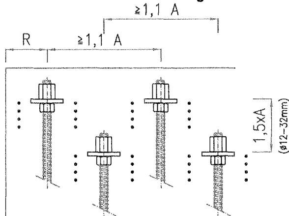
versetzte Verankerung
