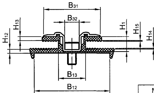
Oberer Klemmgummi
