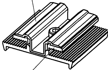
Oberer Klemmgummi
