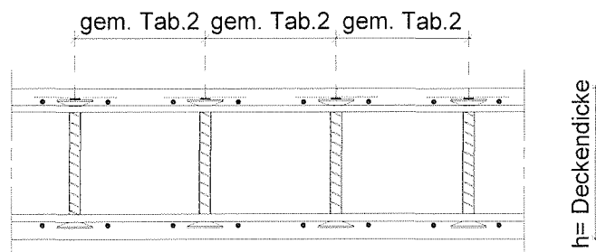
Schnitt B-B
