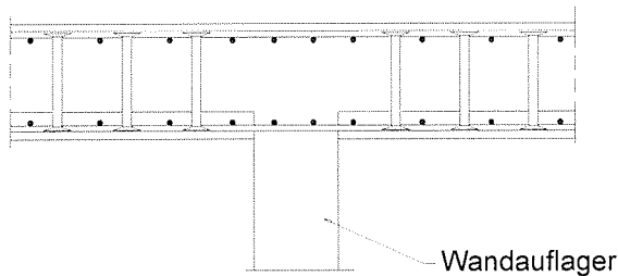
Beispiel 4: Elementdecke
