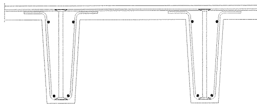
Beispiel 3: TT- Platte
