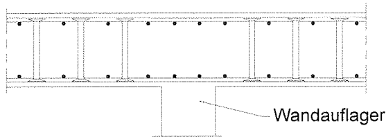
Beispiel 1: Platte
