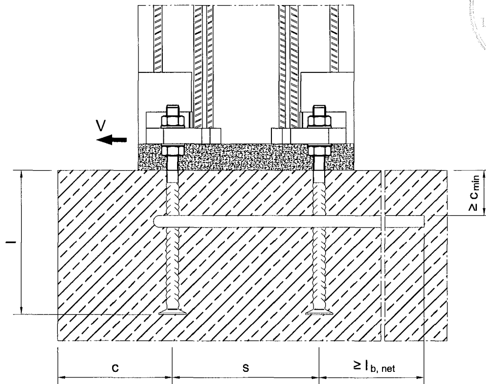
Bild 15: Konstruktive Ausbildung der Rückhängebewehrung
