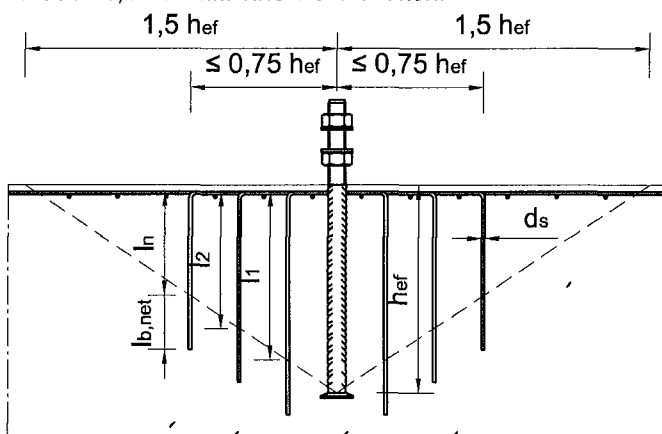
Bild 8: Beispiel für die Ausbildung der Rückhängebewehrung, bei der die Bemessung einer Oberflächenbewehrung erforderlich ist
