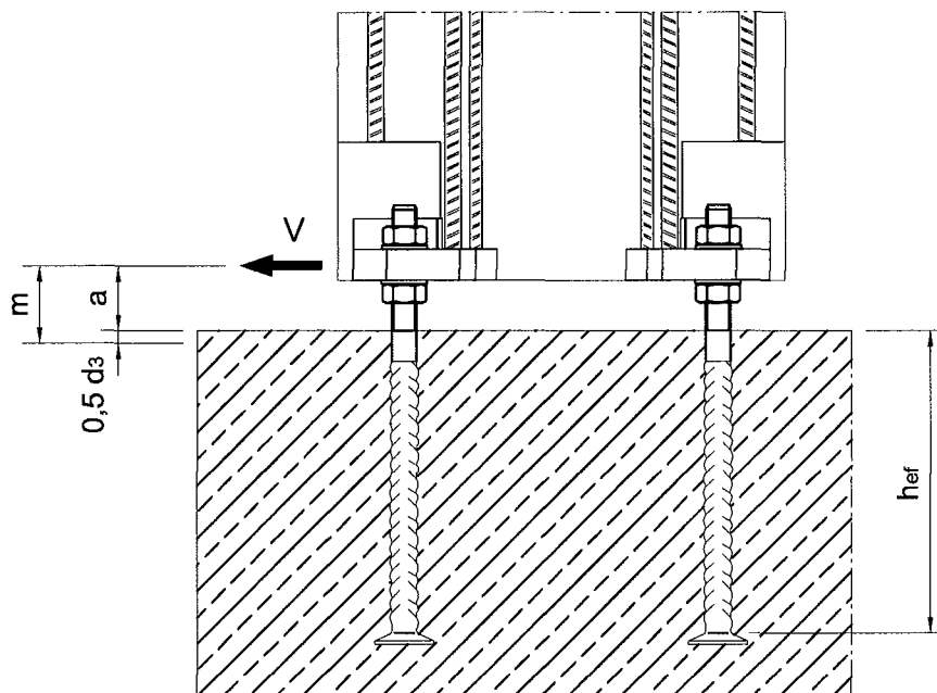
Bild 9: Festlegung des Hebelarms
