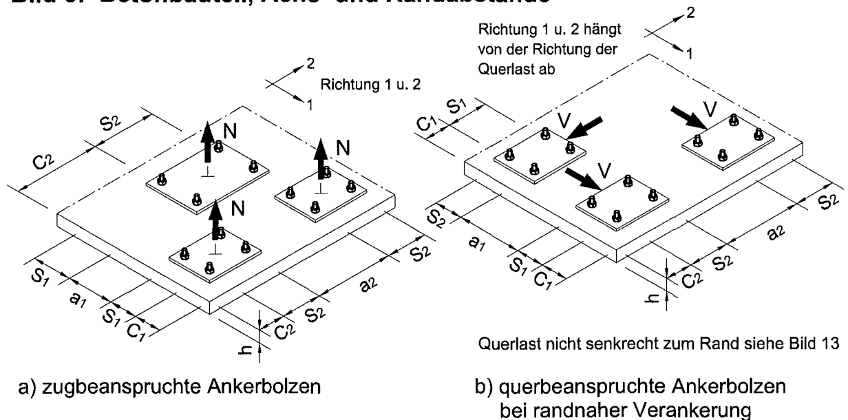
Bild 3: Betonbauteil, Achs- und Randabstände
