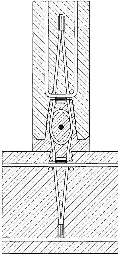
Bild 14: Wand - Wand - T-Verbindung
