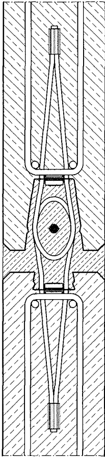
Bild 13: Wand - Wandverbindung
