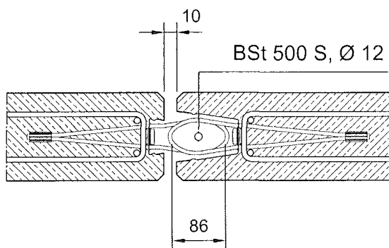
Bild 9: Minimale Fuge
