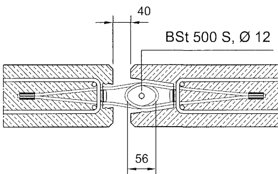
Bild 10: Maximale Fuge
