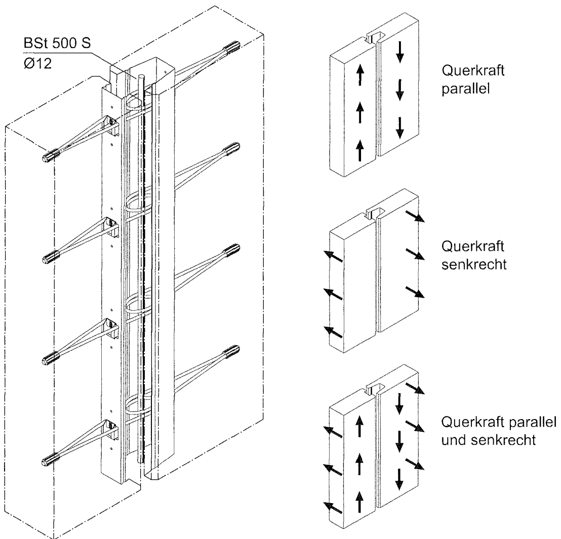
Bild 3: Einbauzustand ohne Fugenverguss und zulässige Belastungsrichtungen
