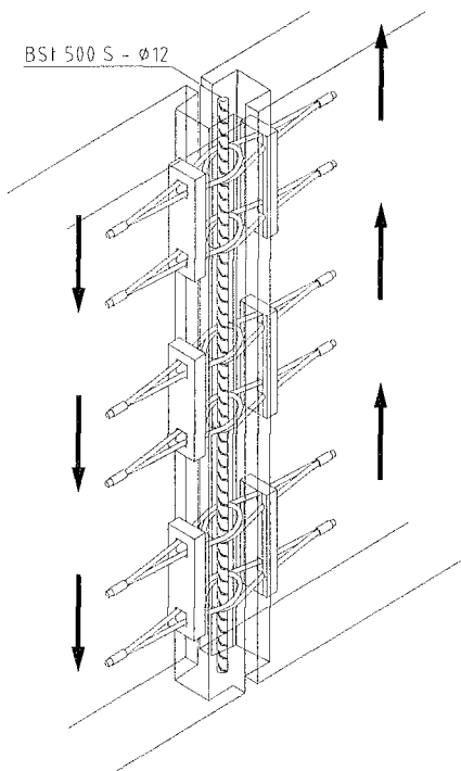
Bild 9: Beanspruchung parallel zur Fugenlängsrichtung
