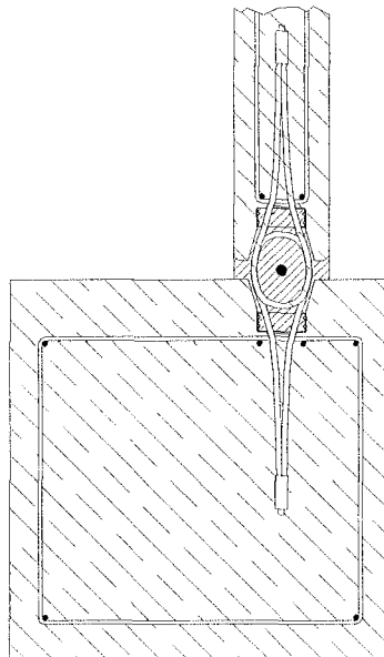
Bild 4: Stützen - Wandverbindung
