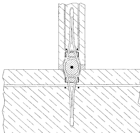
Bild 7: Wand – Wand – T-Verbindung - Regeldetail
