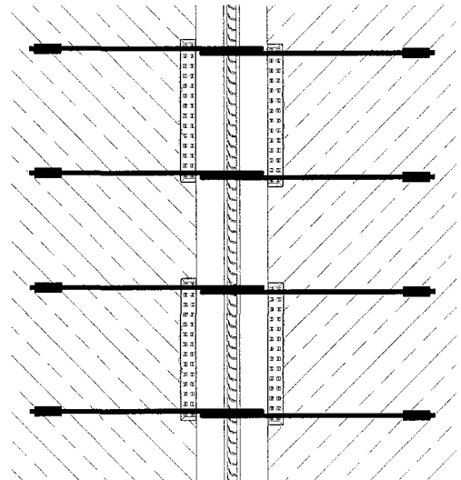
Bild 16: Regelfall Schlaufenüberlappung
