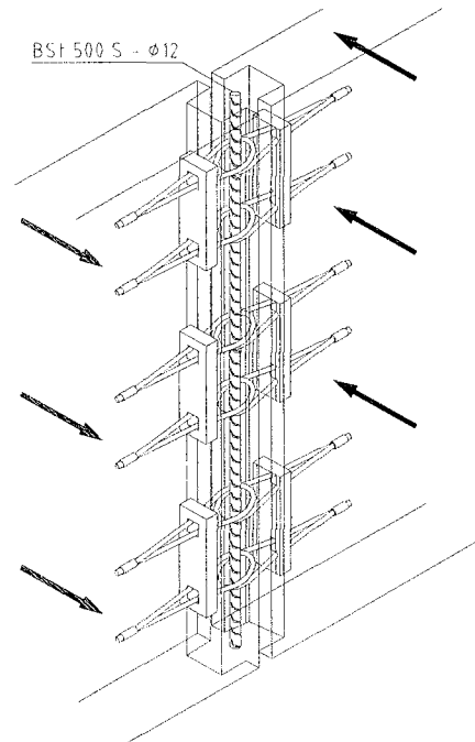
Bild 10: Beanspruchung senkrecht zu Fugenlängsrichtung und Wandebene
