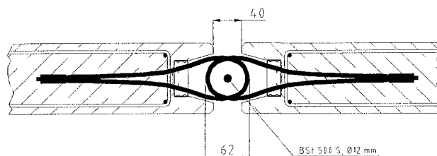
Bild 15: Maximale Fuge
