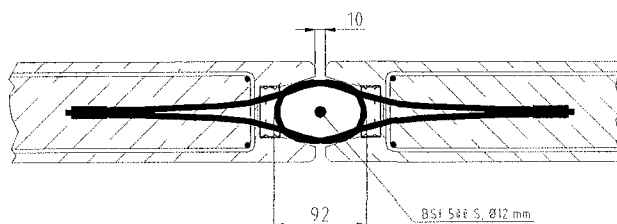
Bild 14: Minimale Fuge
