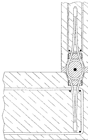
Bild 5: Wand – Wand – Eckverbindung - Regeldetail
