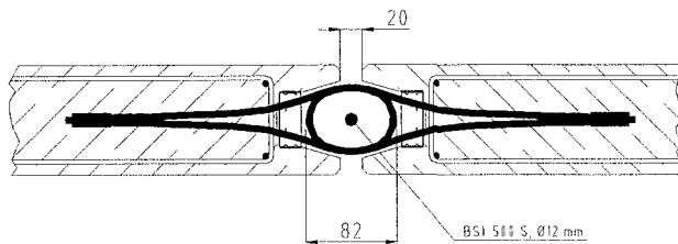
Bild 13: Regelfall Fuge
