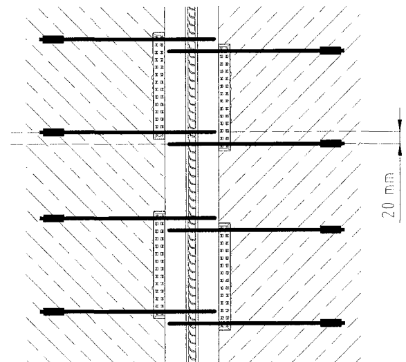
Bild 17: Maximale vertikale Fehllage: 20 mm
