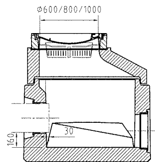
Probenahmeschacht als Probenahmeverrichtung gemäß DIN 1999-100
