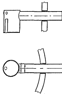
Probenahmebehälter
