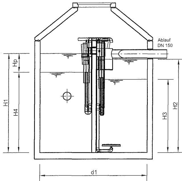
Schnitt A-A
