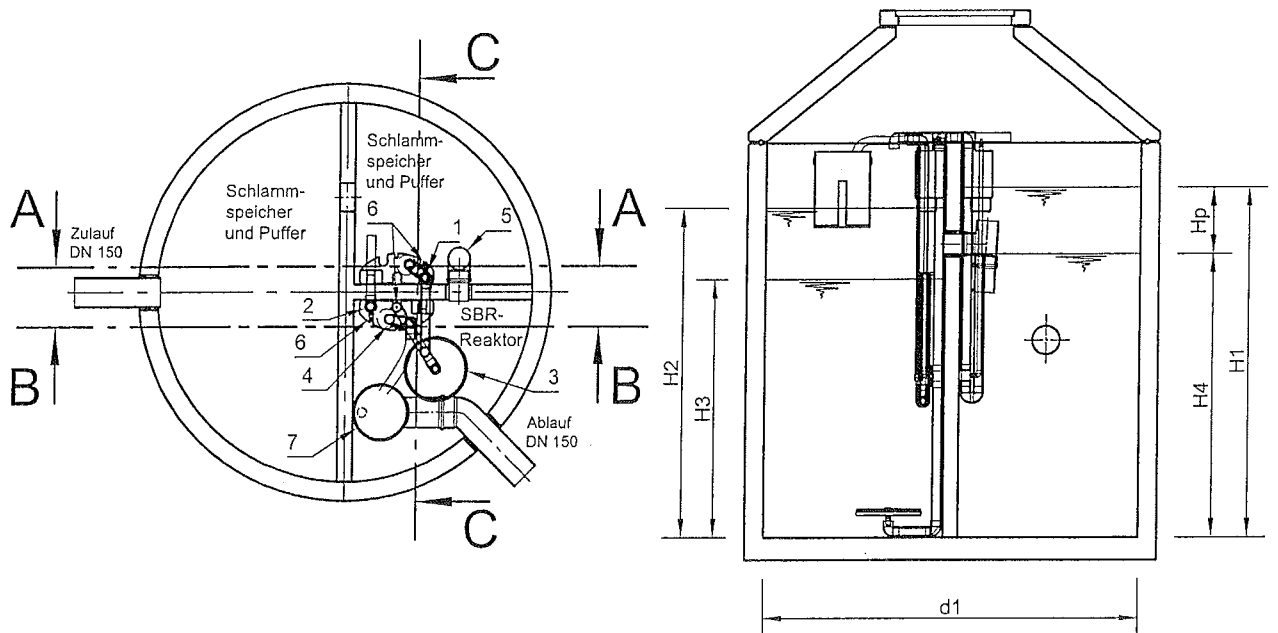
Schnitt C-C
