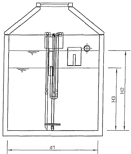
Schnitt C-C
