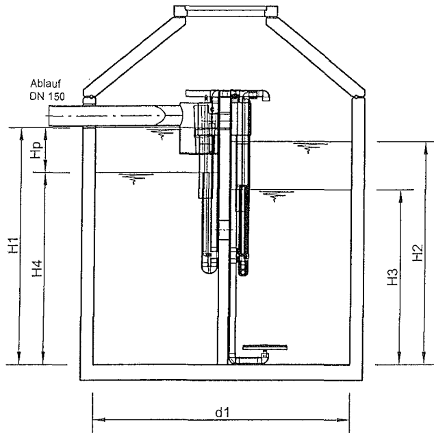
Schnitt A-A
