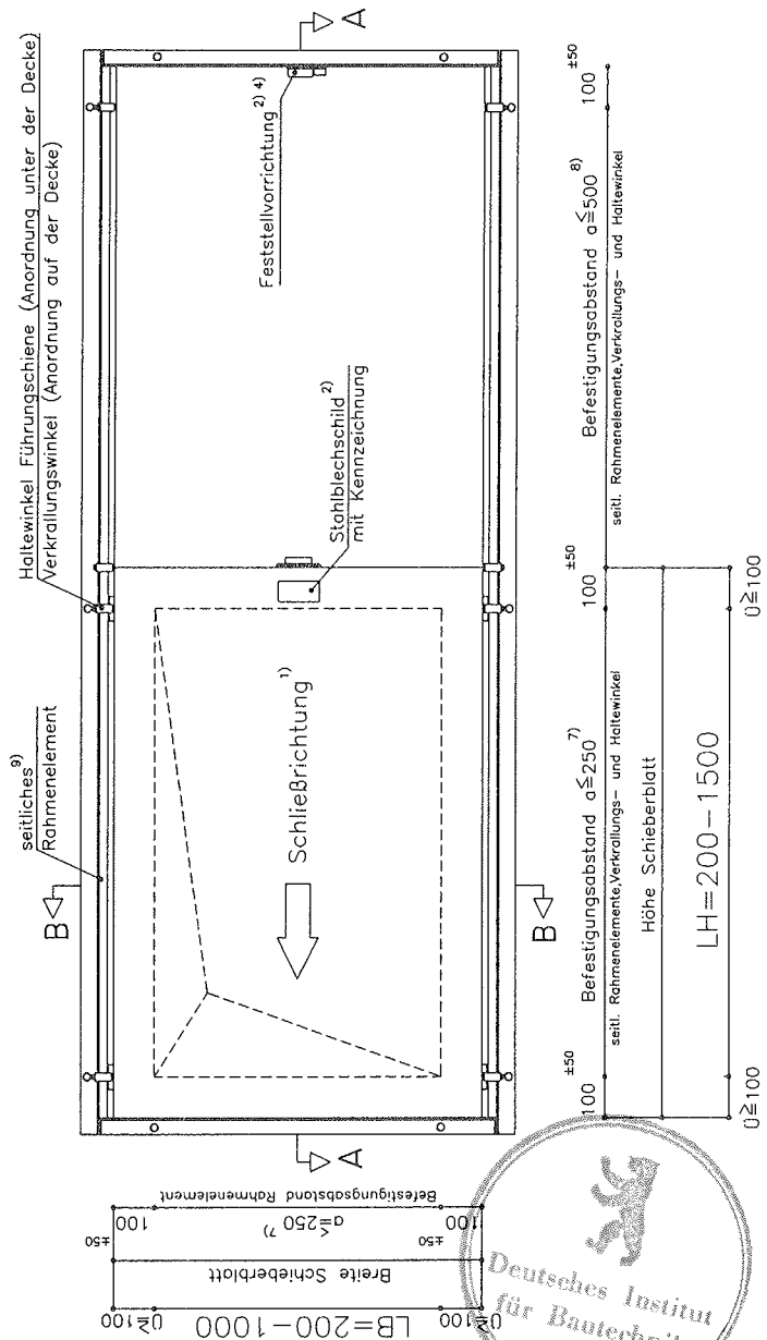
VORDERANSICHT
