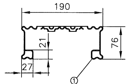
Querschnitt
