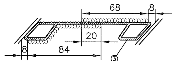
Verschweißung der Stufen im Detail
