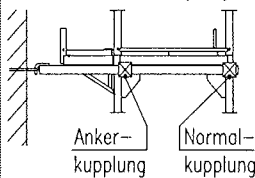
V-Anker
