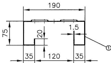
Querschnitt
