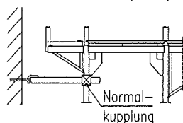
Gerüsthalter (KV2)
