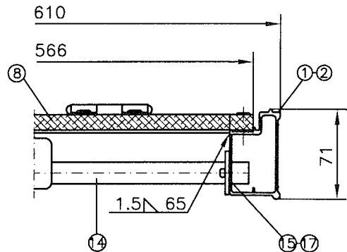
Schnitt B-B
