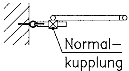
Bild B.2a: Gerüsthalter
