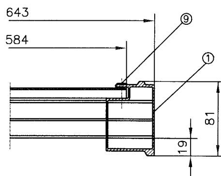
Schnitt A-A
