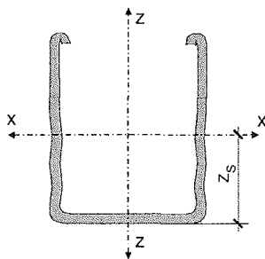
Bild 4: Kennwerte des oberen Querriegels im Bereich der Belagsicherung
