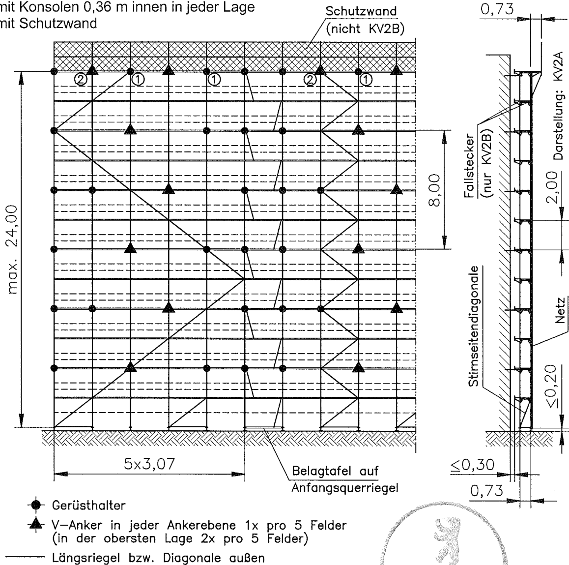
Gerüsthalter (GV)
