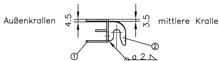
Schnitt A-A
