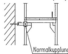
Gerüsthalter (KV2)
