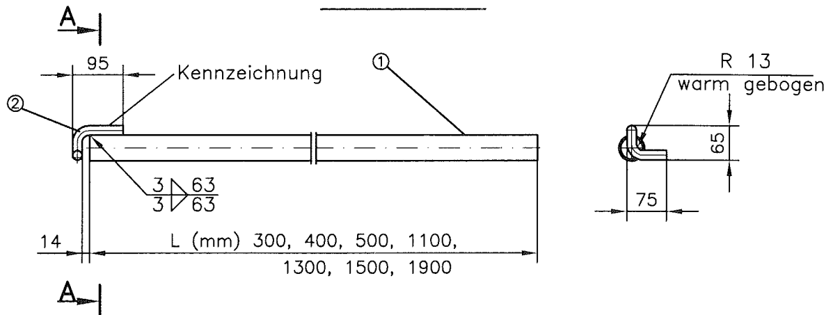
Schnitt A-A
