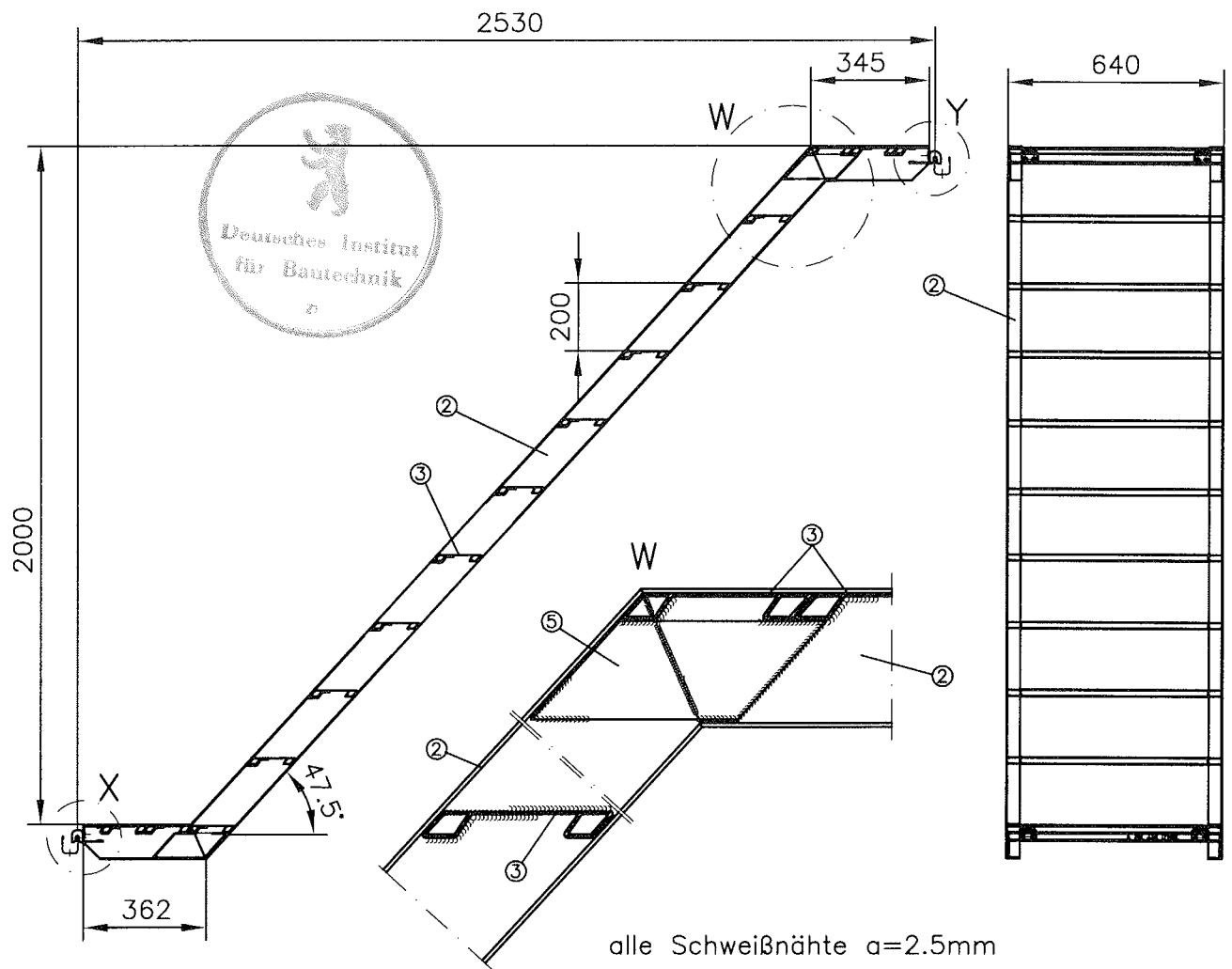
Verschweißung der Stufen im Detail
