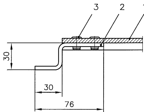
Schnitt A-A
