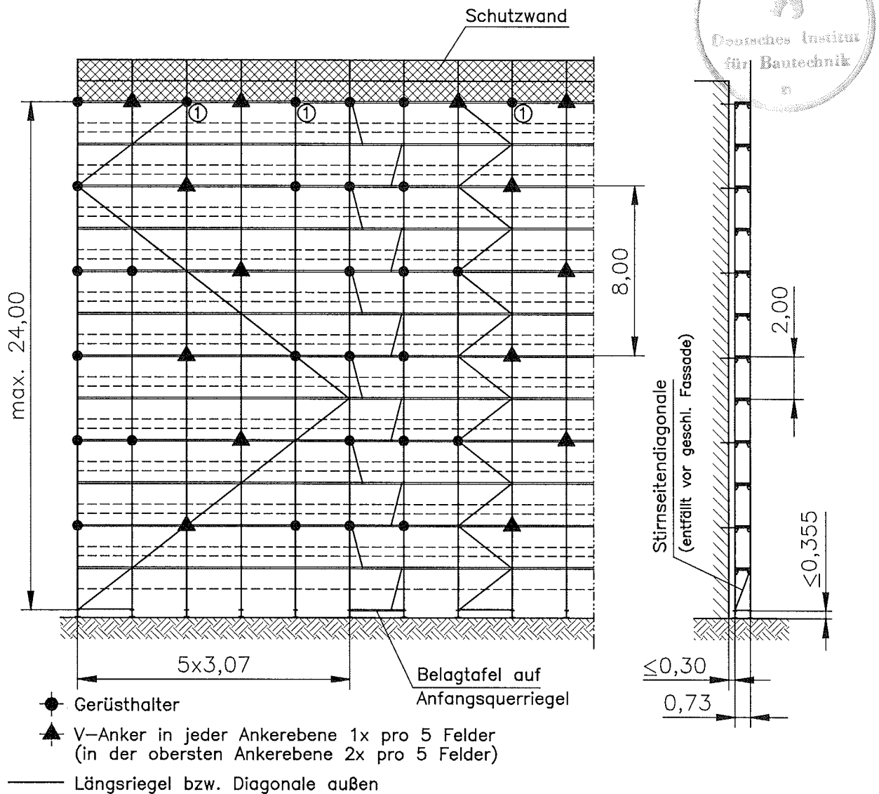
Gerüsthalter (GV)
