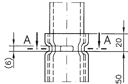
Detail X Rohrverbindung durch Einpressen
