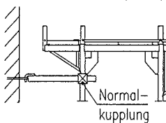
Gerüsthalter (KV2)
