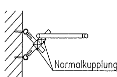
V-Anker
