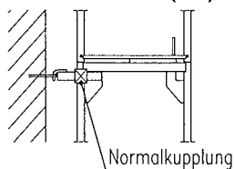
Gerüsthalter (KV2)
