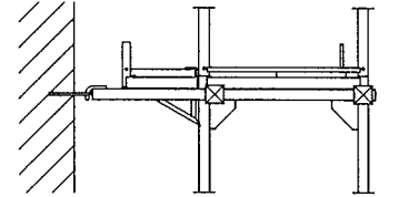
Gerüstlage mit Konsolen
