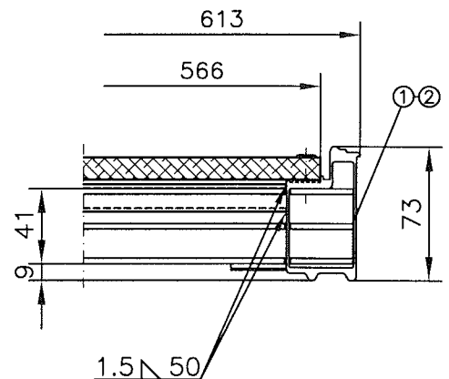
Schnitt A-A
