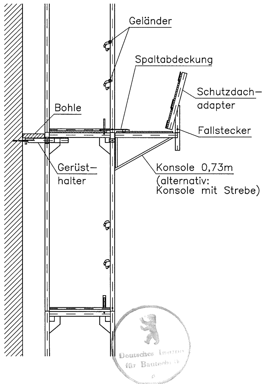
Bild B.5: Schuttdach mit Konsolen 0,73 m und Schuttdachadaptern
