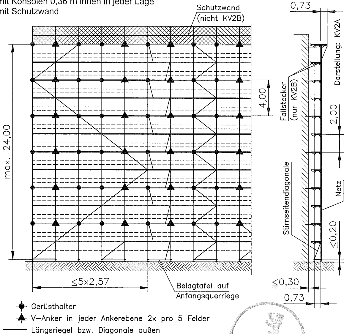
Gerüsthalter (GV)
