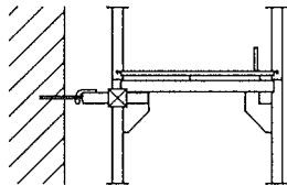
Gerüstlage ohne Konsolen
