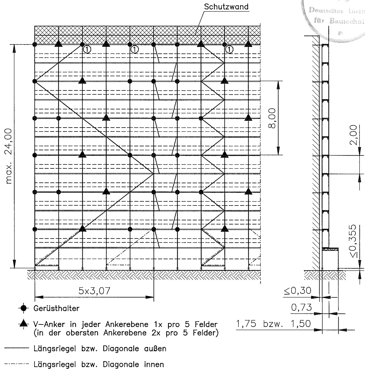
Gerüsthalter (GV)
