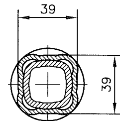
Schnitt A-A
