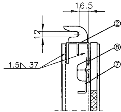
Schnitt A-A
