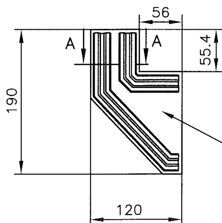
Knotenblech
