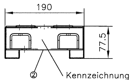
Kopfbeschlagn
