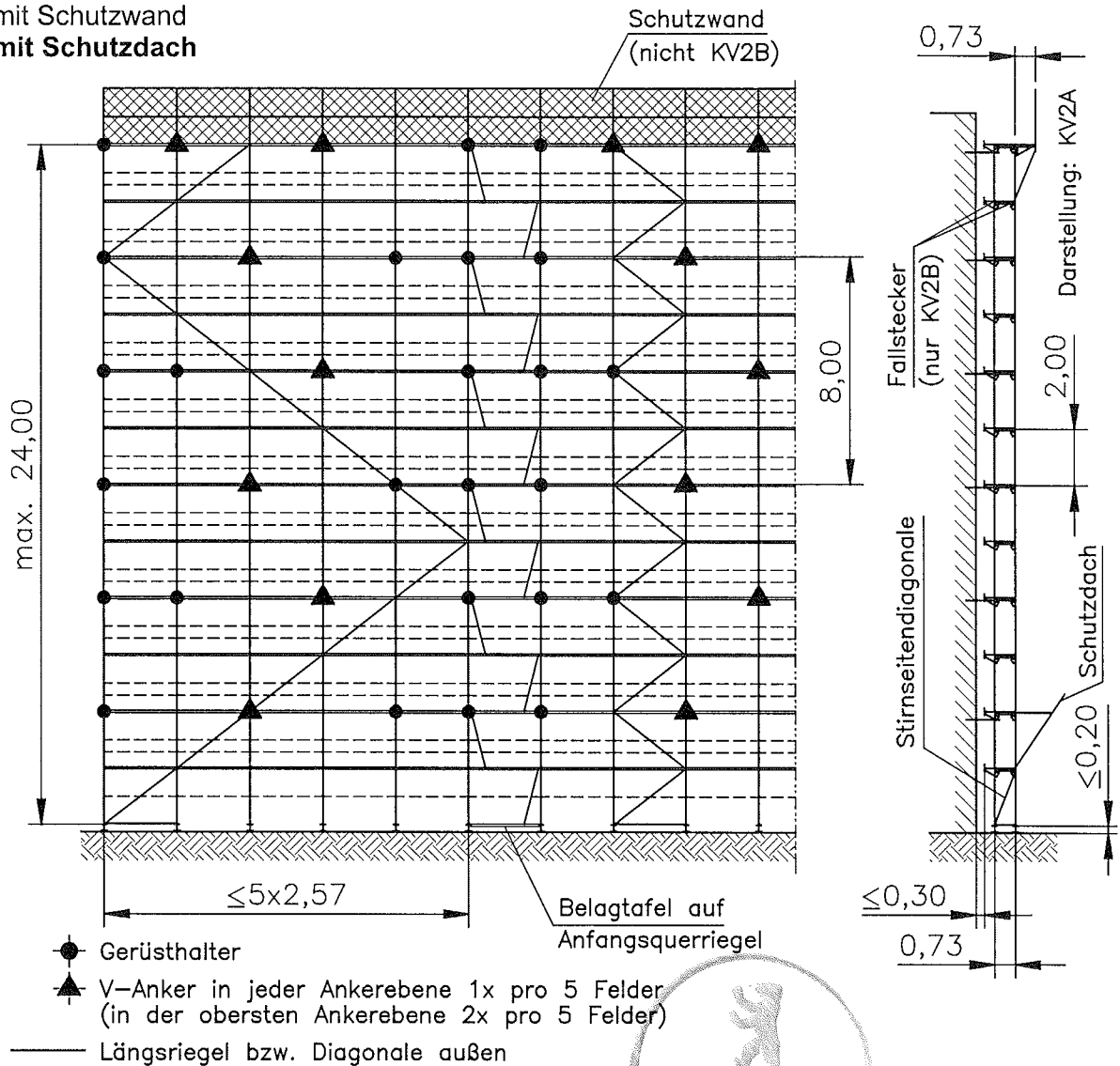
Gerüsthalter (GV)
