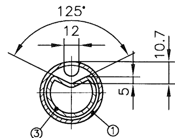
Schnitt A-A
