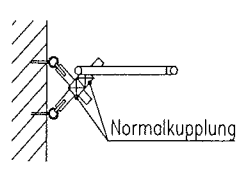
V-Anker
