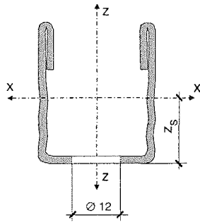
Bild 3: Kennwerte des oberen Querriegels mit Lochung
