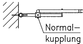
Bild B.2b: Schnellanker
