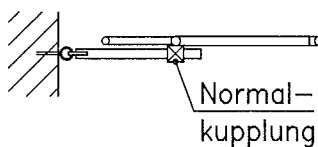
Bild B.2d: Gerüsthalter
