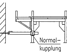
Gerüsthalter (KV2)
