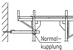
Gerüsthalter (KV2)
