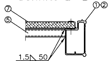
Schnitt B-B
