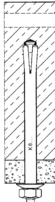
Durchsteckmontage Außengewinde
