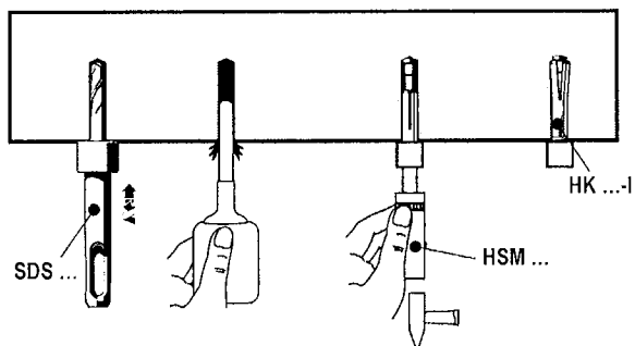
Setzen des HK ...-I mit Handsetzwerkzeug
