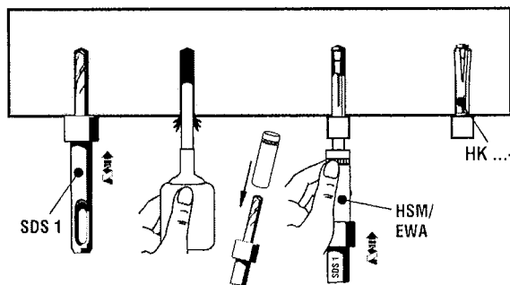
Setzen des HK ...-I mit Maschinensetzwerkzeug
