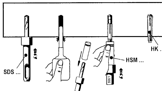
Setzen des HK mit Maschinensetzwerkzeug
