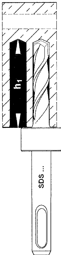
Bundbohrer SDS 2
