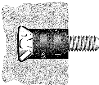
Bündigmontage (Carbonhülse)
