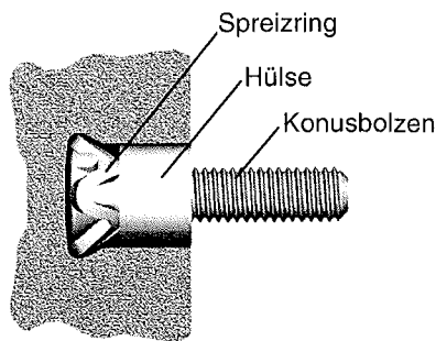
Bündigmontage (Stahlhülse)
