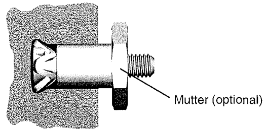
Abstandsmontage (Stahlhülse)
