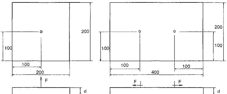
Bild 6: zentrischer Zug bzw. Querzug für einen Randabstand 100/100 mm
