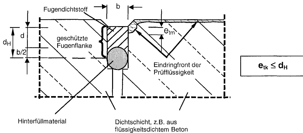
Bild 1: Umläufigkeitsverhalten im Bereich des eingebauten Fugenabdichtungssystems 1)
