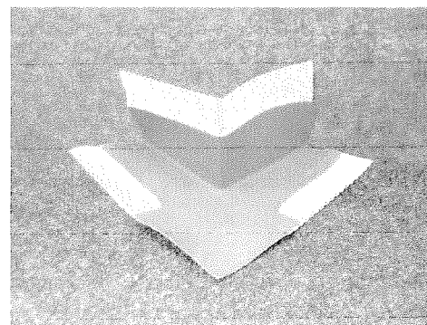
Außeneckendichtung "KÖSTER BD 72 Flex-Band Außenecke"
