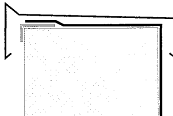
Abb. 14: Dachrandabschluss mit Mauerabdeckprofilen
