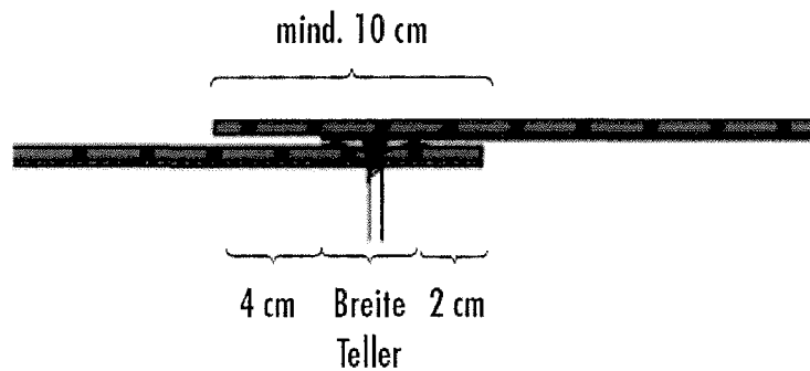
Abb.1: Mindestüberlappungen im Längsnahtbereich Abstand der Bahnenkante der unteren Bahn vom Rand des Befestigers mindestens 2 cm
