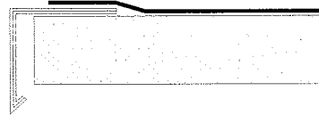
Abb.11: Dachrandabschluss mit Verbundblech-Traufprofil mit Abkantungen
