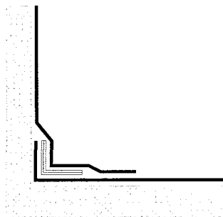
Abb. 5: Anschluss und Kehlausbildung bei lose verlegter Anschlussbahn
