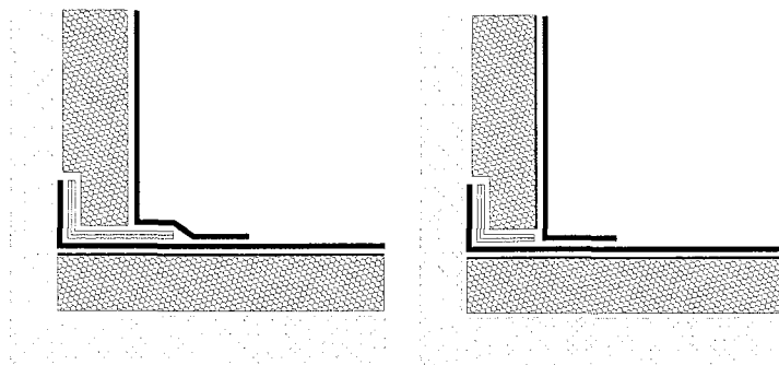
Abb. 6: Anschluss und Kehlausbildung bei wärmegeämmten Bauteilen und lose verlegter Anschlussbahn (linke Darstellung) bzw. bei verklebter Anschlussbahn (rechte Darstellung)
