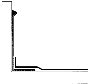
Abb. 3: Anschluss und Kehlausbildung bei Verwendung von Verbundblechprofilen
