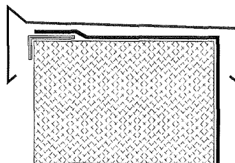
Abb. 14: Dachrandabschluss mit Mauerabdeckprofilen
