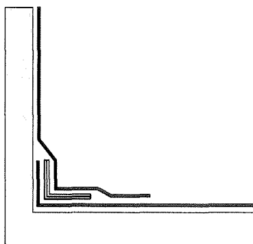
Abb. 4: Anschluss und Kehlausbildung bei verklebter Anschlussbahn
