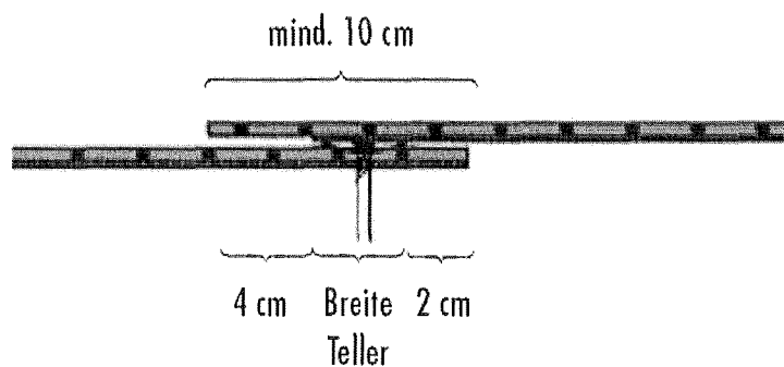
Abb.1: Mindestüberlappungen im Längsnahtbereich Abstand der Bahnenkante der unteren Bahn vom Rand des Befestigers mindestens 2 cm
