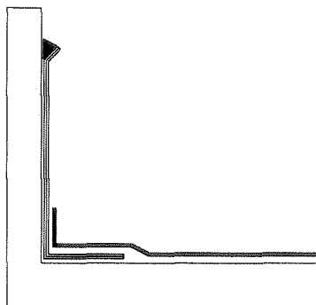
Abb.3: Anschluss und Kehlausbildung bei Verwendung von Verbundblechprofilen
