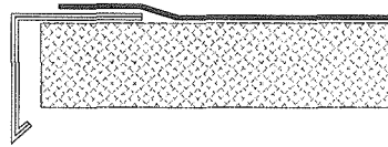
Abb.11: Dachrandabschluss mit Verbundblech-Traufprofil mit Abkantungen
