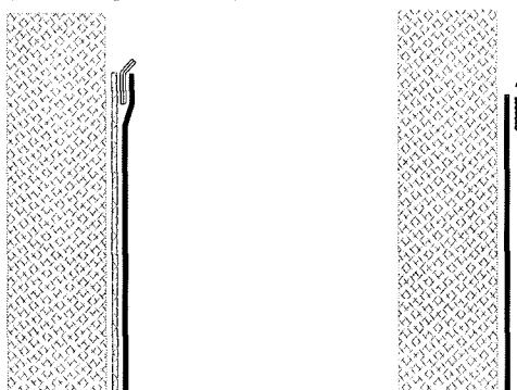
Abb. 10: Obere Verwahrung mit Verbundblech (linke Darstellung) bzw. mit Klemmprofil (rechte Darstellung)
