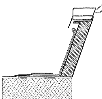
Abb.15: Einfassung von Lichtkuppel-Aufsetzkränzen mit Verbundblechprofilen
