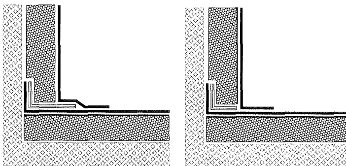
Abb. 6: Anschluss und Kehlausbildung bei wärmegeädämmten Bauteilen und lose verlegter Anschlussbahn (linke Darstellung) bzw. bei verklebter Anschlussbahn (rechte Darstellung)
