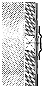
Abb. 8: Zwischenbefestigung an aufgehende gedämmte Bauteile mit Holzbohle und Verbundblech
