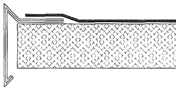
Abb. 12: Dachrandabschluss mit Verbundblechprofil
