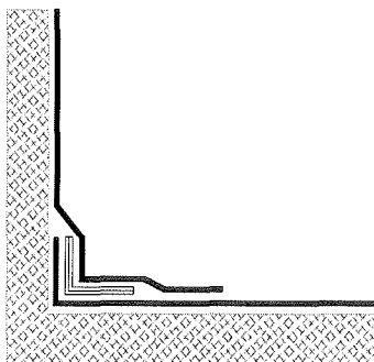
Abb. 5: Anschluss und Kehlausbildung bei lose verlegter Anschlussbahn
