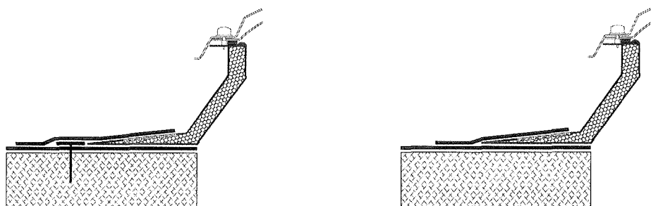
Abb. 17: Einfassung von Lichtkuppel-Aufsetzkränzen mit Hart-PVC-Rahmen, mit Kehlbefestigung (linke Darstellung) bzw. ohne Kehlbefestigung (rechte Darstellung)
