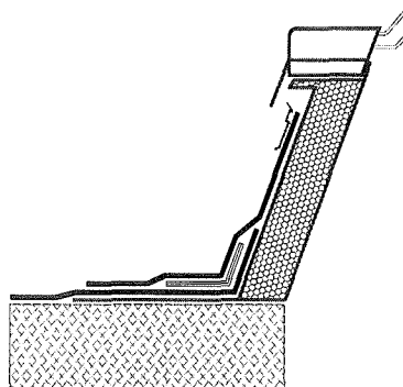
Abb. 16: Einfassung von Lichtkuppel-Aufsetzkränzen mit Bahnenstreifen
