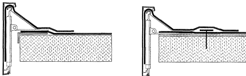
Abb. 13: Dachrandabschluss mit mehrteiligen Metall-Klemmprofilen, rechte Darstellung bei vorhandenen mehrteiligen Metallprofilen
