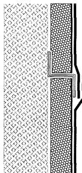
Abb. 9: Zwischenbefestigung an aufgehende gedämmte Bauteile mit Verbundblech (Z-Profil)
