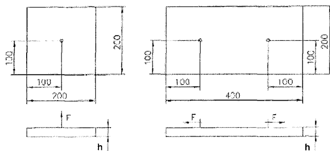
Bild 1: Versuchskörper zentrischer Zug und Querkzug
