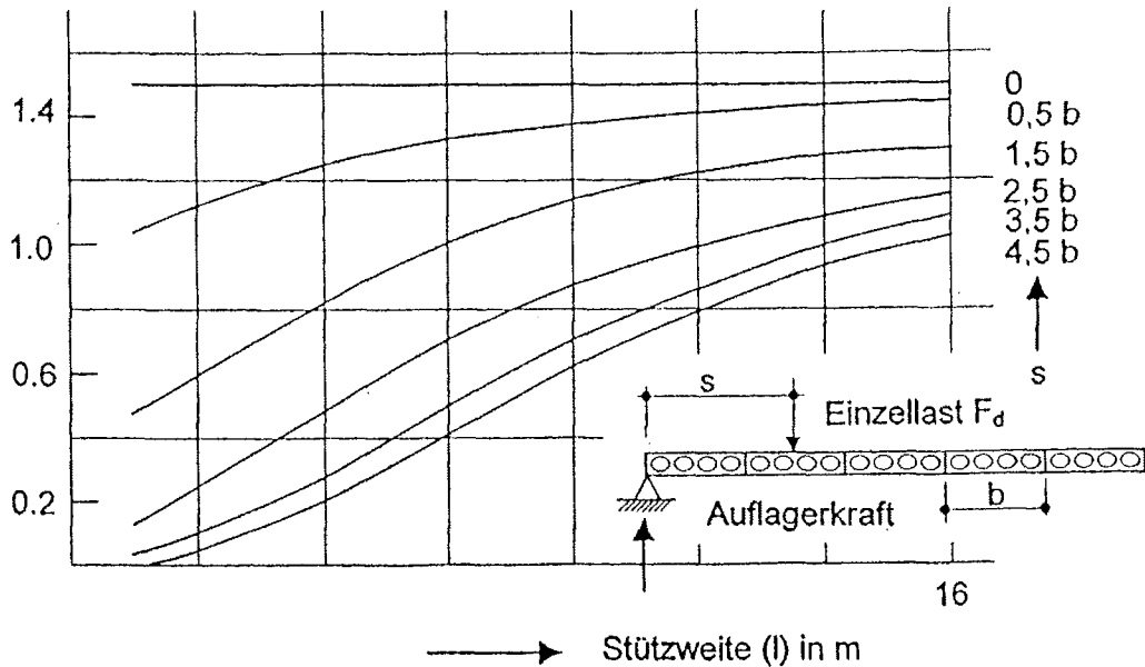
Auflagerkraft am Längsrand infolge Einzellast in Feldmitte
