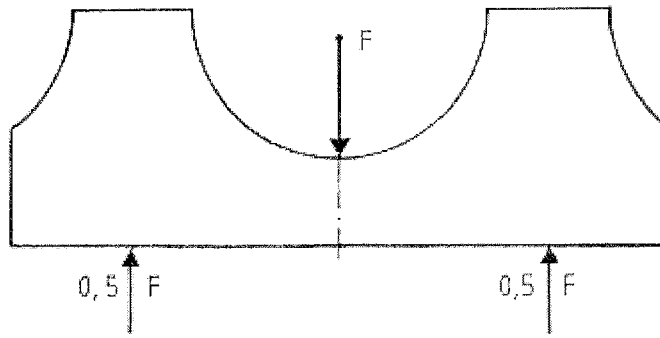
Bild 1: Belastungsanordnung Biegeversuch
