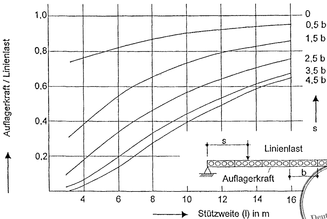
Auflagerkraft am Längsrand infolge Linienlast
