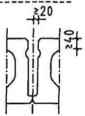
Fugedetail
