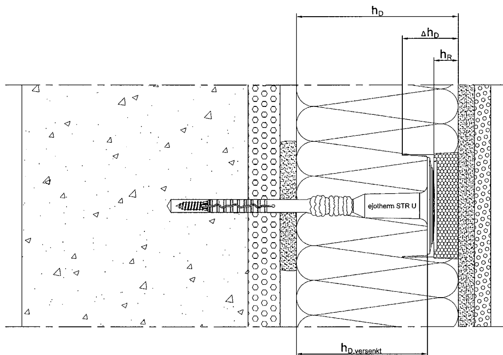
Bild 5.1: ejotherm STR-U (versenkte Montage)
