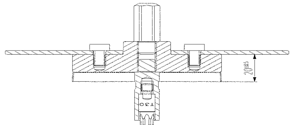
Bild 4.2: EJOT ejotherm Montagetool Typ "S" für Dämmstoffdicken ab 80 mm
