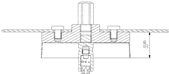
Bild 4.1: EJOT ejotherm Montagetool Typ "L" für Dämmstoffdicken ab 100 mm
