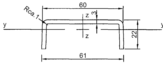
U-Profil: 60/22/3
