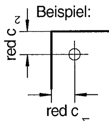
Bild 6: Reduzierte Randsabstände
