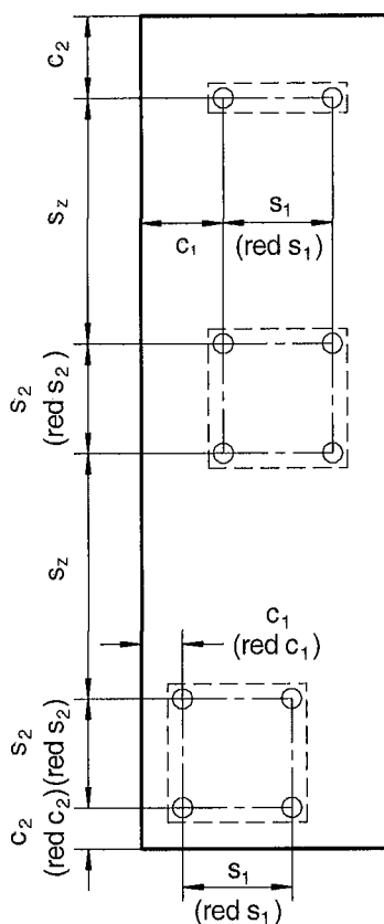
Bild 7: Gewindehülsegruppen
