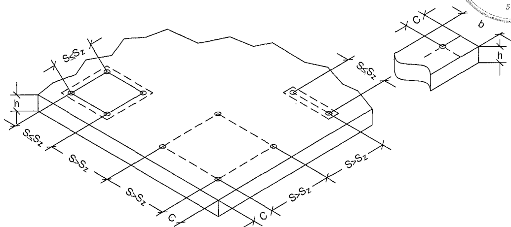
Bild 5: Bezeichnung der Abstände und Abmessungen
