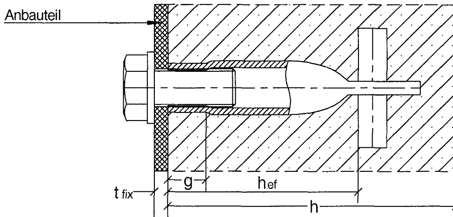
Bild 2: Schroeder-Gewindehülse mit angeschweißter Nagelplatte
