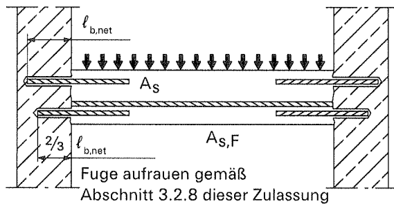
Endverankerung von Platten oder Balken
