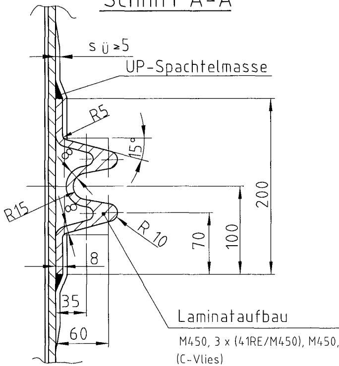
Schnitt A-A
