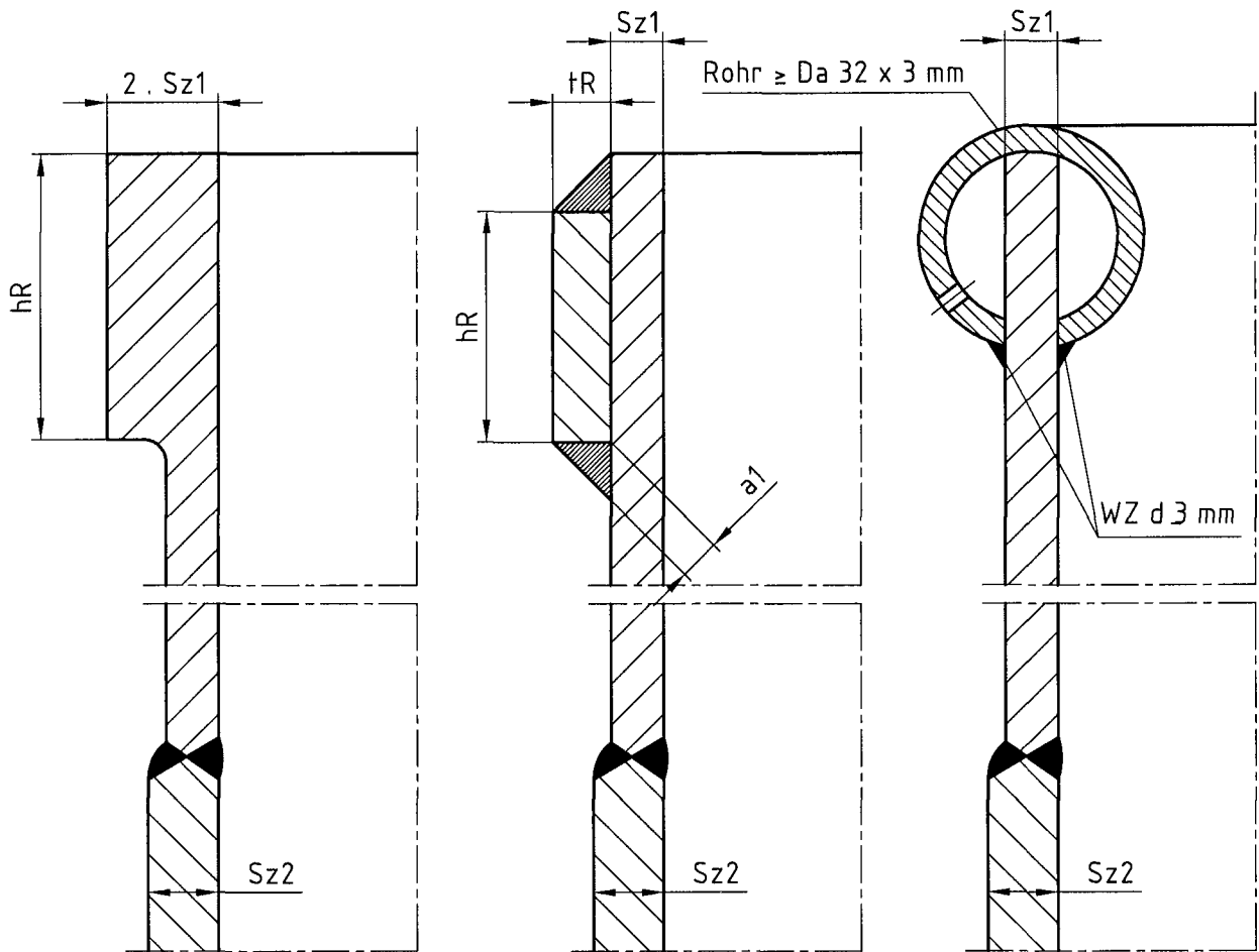
mit Verstärkungsring
