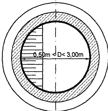
Schachtquerschnitt: rund oder eckig
