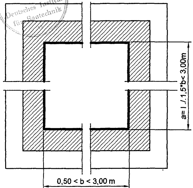
Schachtquerschnitt: rund oder eckig
