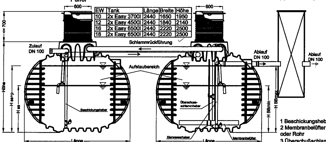
Schlamm-speicher Puffer SBR-Reaktor
